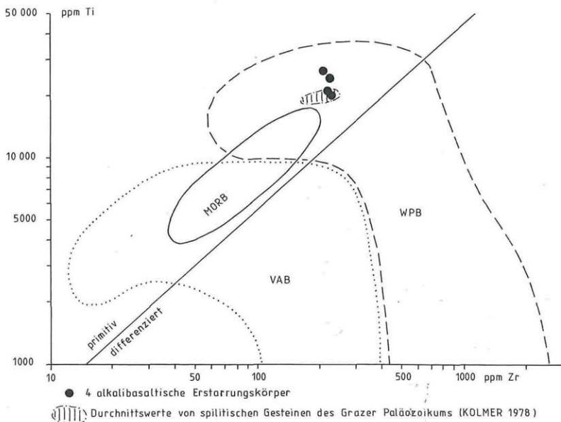
Abb. 5: Ti-Zr-Diagramm nach PEARCE (1983) für 4 Spilite aus dem Grazer Paläozoikum. Die Werte sind H_2O^+ - und CO_2 -frei berechnet. Zum Vergleich sind die von Kolmer (1978) untersuchten spilitischen Gesteine des Grazer Paläozoikums mit eingetragen. MORB = Feld der Basalte mittelozeanischer Rücken, VAB = Feld der Inselbogenlaven, WPB = Feld der Intraplattenlaven.
