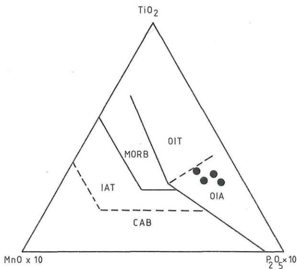
Abb. 6: MnO \times 10 - TiO_2 - P_2O_5 \times 10 -Diagramm nach MULLEN (1983) für 4 Spilite aus dem Grazer Paläozoikum. OIA = Feld der Alkalibasalte ozeanischer Inseln, OIT = Feld der tholeiitischen Basalte ozeanischer Inseln, MORB = Feld der Basalte mittelozeanischer Rücken, IAT = Feld der Inselbogen-Tholeiite, CAB = Feld der Kalkkali-Basalte.
