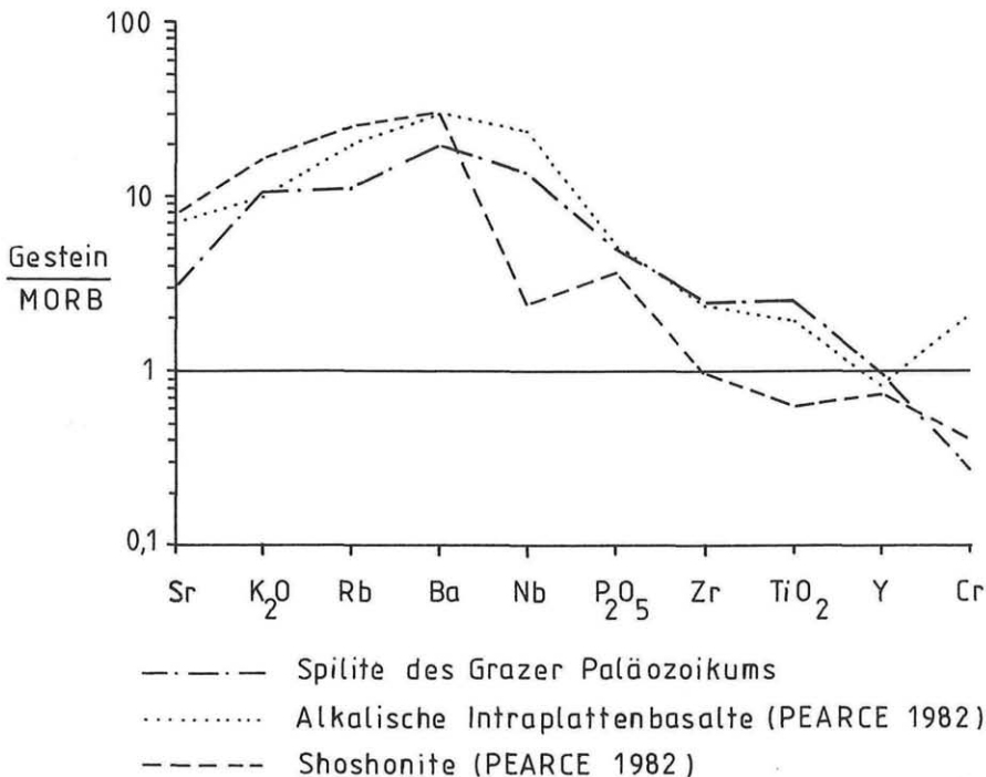
Abb. 7: Durchschnittswerte ausgewählter Haupt- und Spurenelemente von 4 Spiliten aus dem Grazer Paläozoikum, normiert mit entsprechenden Werten mittelozeanischer Rückenbasalte (MORB) nach PEARCE (1982). Zum Vergleich sind die Verteilungskurven von alkalischen Intraplatten-Basalten und Shoshoniten nach PEARCE (1982) mit eingetragen.
