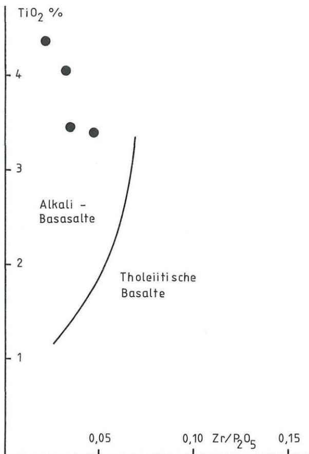
Abb. 2: TiO 2 -Zr/P 2 O 5 -Diagramm nach FLOYD & WINCHESTER (1975) für 4 Spilite aus dem Grazer Paläozoikum. Die TiO 2 -Werte sind H 2 O + - und CO 2 -frei berechnet.
