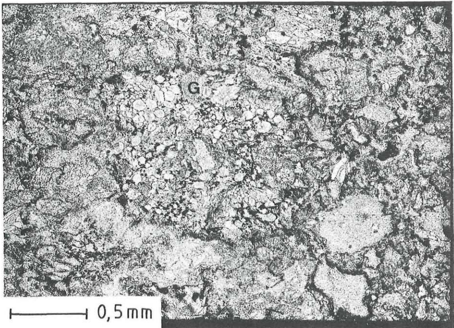
Abb. 3: Dünnschliff-Photographie einer pyroklastischen Lage aus dem Givet des Grazer Paläozoikums (Lokalität: Rote Wand, südwestlich des Hochlantsch). G = chloritisierte ehemals basaltische Glasscherben, die zahlreiche Bläschen führen.
