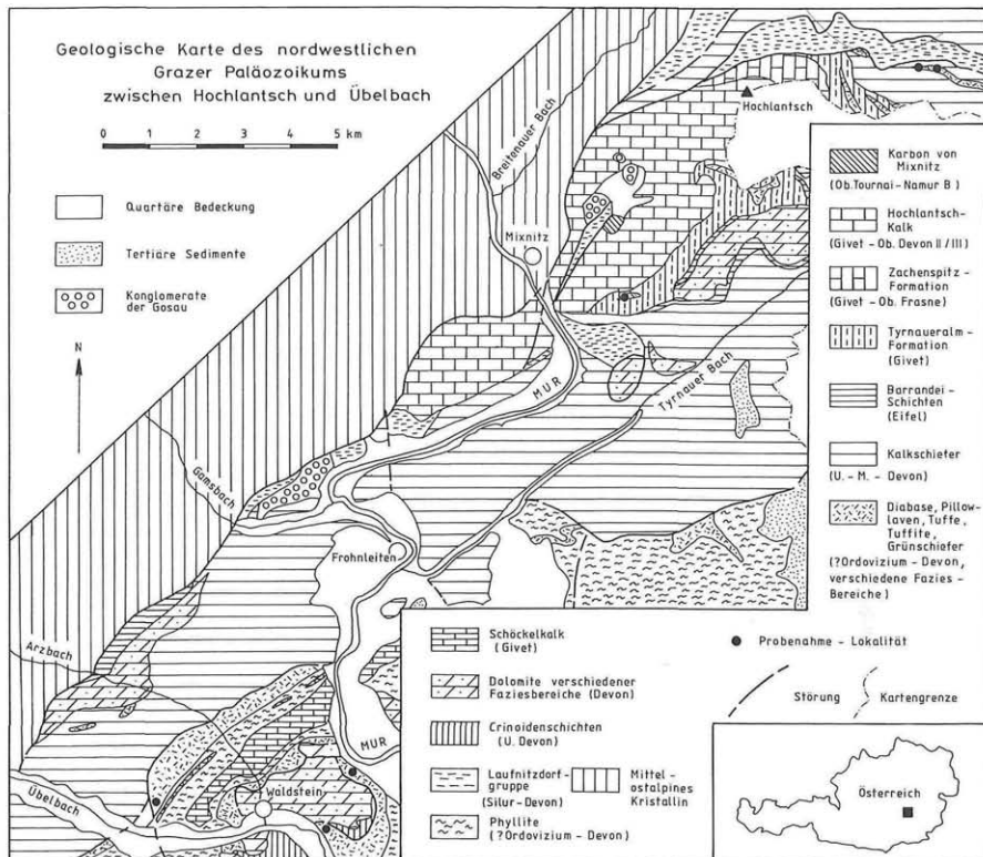
Abb. 1: Vereinfachte geologische Karte des nordwestlichen Grazer Paläozoikums zwischen Hochlantsch und Übelbach nach EBNER et al. (1983), die die Probenahme-Lokalitäten zeigt.
