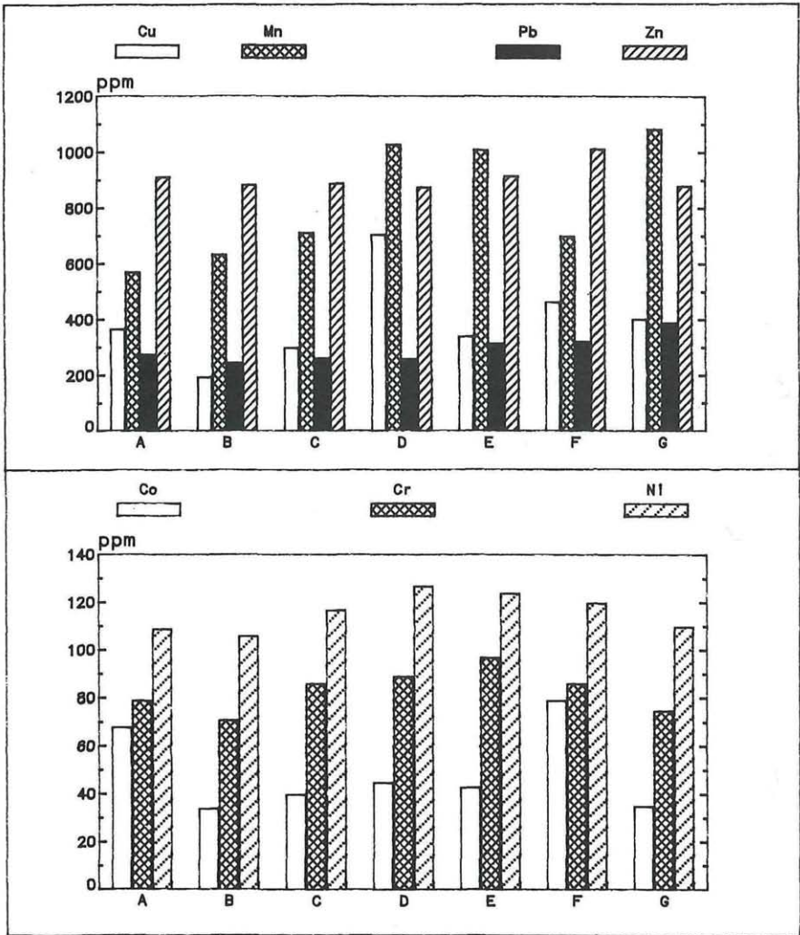
Abb. 7: Schwermetallgehalte der Sammelproben A–G. Cu in den Sedimenten des Stromstriches erhöht; Sedimente des Schleusenbereiches zeigen generell niedrigere Schwermetallgehalte.
