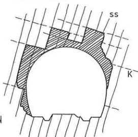
Abb. 4: Ausbruchsformen und Überprofiltypen im Plabutsch-Tunnel (Typus 7-12a)
