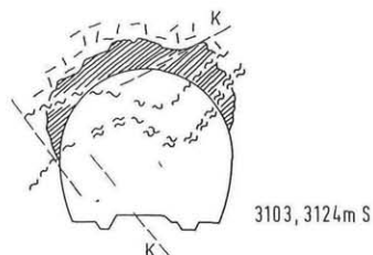
Abb. 5: Ausbruchsformen und Überprofiltypen im Plabutsch-Tunnel (Typus 12b-15)
