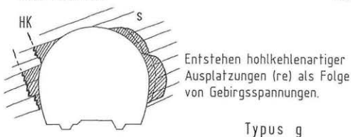
Abb. 2: Überprofiltypen im Gleinalm-Tunnel
