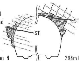
Abb. 4: Ausbruchsformen und Überprofiltypen im Plabutsch-Tunnel (Typus 7-12a)
