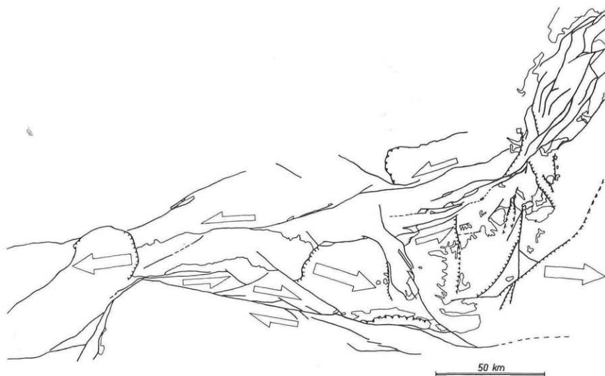
Abb. 6: Dehnungstektonik im Jungtertiär. Das Störungs- und Abschiebungsmuster der Zentralalpen. Dicke Linien: Seitenverschiebungen; Linien mit Zähnen: Abschiebungen.
