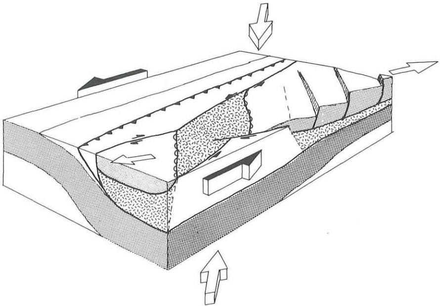
Abb. 10: Schematisches Transpressionsmodell für Gebirgsbildung, um finale orogenparallele Strukturen von Gebirgen zu erklären. Schräge Kollision wird aufgelöst in eine seitenverschiebende und eine orthogonale Bewegungskomponente.
