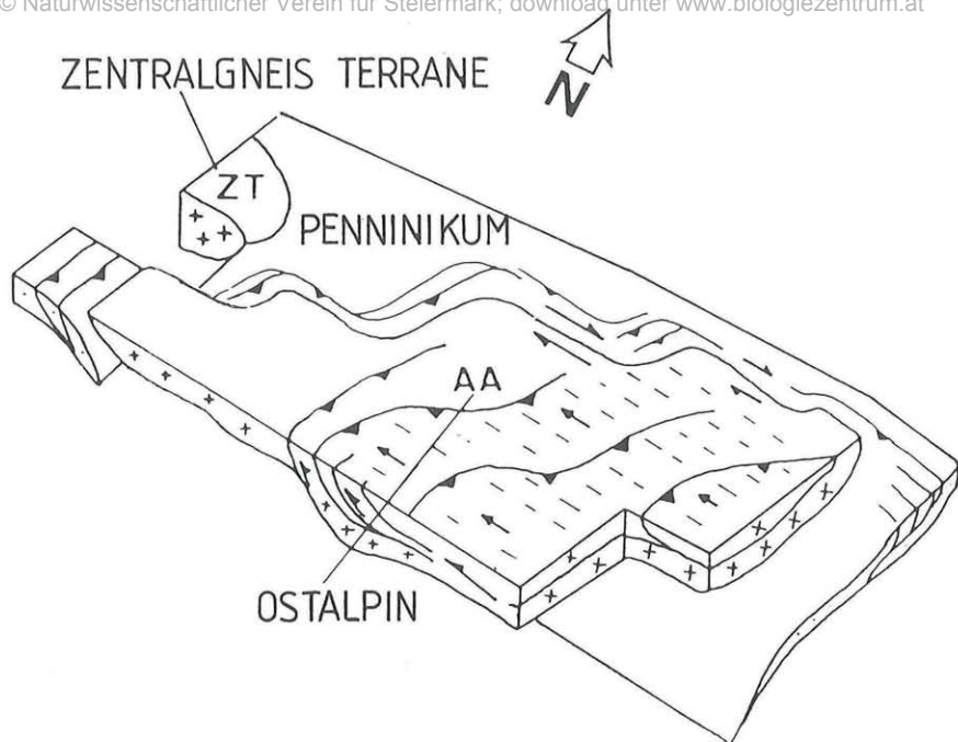
Abb. 3: Transpressive, nordwest- und westgerichtete Überschiebungstektonik und Imbrikation des Ostalpins während der Unter- und Mittelkreide (nach RATSCHBACHER et al., 1989).
