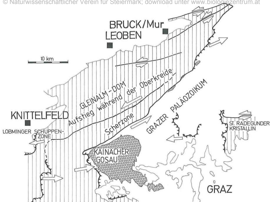
Abb. 5: Krustendehnung, Aufstieg des Metamorphosedomes der Gleinalm und Absinken des Sedimentationsbeckens der Kainacher Gosau während der Oberkreide. Dicke Linien: Störungen; dicke Linien mit Zähnnchen bedeuten Abschiebungen.
