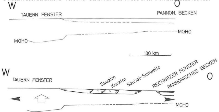
Abb. 7: Profile zu einem Modell der Ausdünnung der Kruste im Jungtertiär. a – Tiefenlage der Moho auf Grund geophysikalischer Daten (nach ARIC et al., 1987); b – Interpretation der Oberflächenstrukturen der östlichen Ostalpen, die im wesentlichen durch großräumige Abschiebungen zur Krustendünnung geführt haben. Schwarz: asymmetrische, jungtertiäre Sedimentationsbecken.
