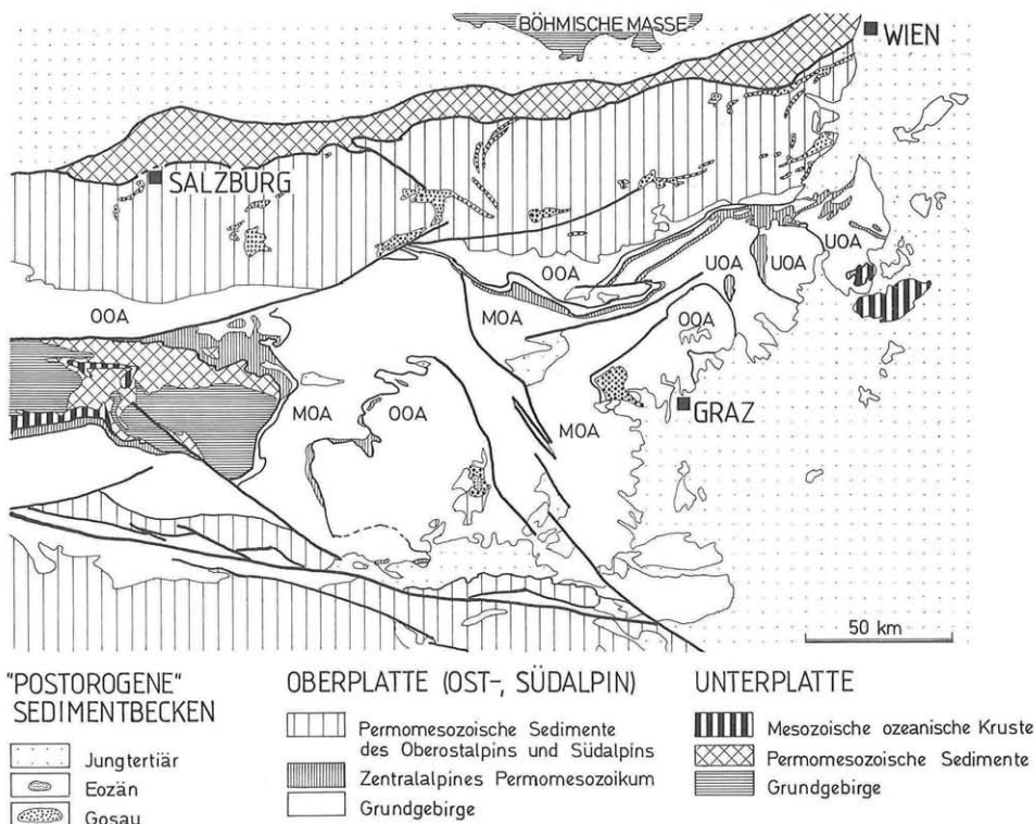
Abb. 2: Vereinfachte tektonische Übersichtskarte der Ostalpen. Die Eozänbecken auf Gosaubecken der Nördlichen Kalkalpen sind weggelassen. UOA – Unterostalpine Deckeneinheiten, MOA – mittelostalpine Deckeneinheiten, OOA – oberostalpine Deckeneinheiten.
