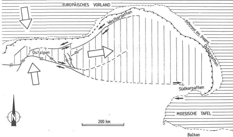
Abb. 8: Das Zersplittern des Ostalpins und das seitliche Herausdrücken von Keilen des Orogens nach Ost während des Jungtertiärs (nach NEUBAUER, 1988).
