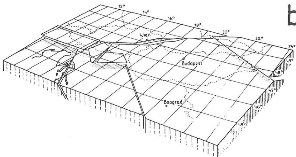
Abb. 9: Verteilung historischer Erdbeben und das daraus abgeleitete blocktektonische Modell (nach GUTDEUTSCH & ARIC, 1987).
