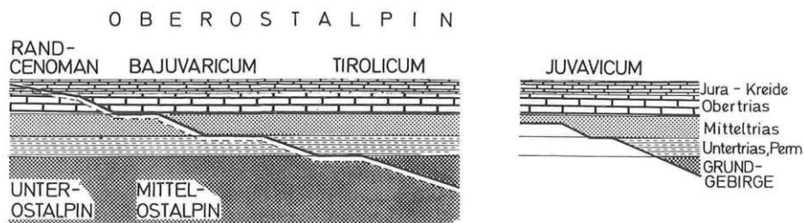
Abb. 4: Schematisches Modell zur Abwicklung und Einwurzelung der Nördlichen Kalkalpen. Bei Annahme einer nordgerichteten Komponente der WNW-Bewegung können die basal unvollständigen Schichtfolgen der Nördlichen Kalkalpen auf die oben amputierten Schichtfolgen des Ostalpins der Zentralalpen gelegt und damit eingewurzelt werden. D. h., größere Bereiche können auf den Zentralalpen eingewurzelt werden. Das Juvavikum benötigt jedoch einen zusätzlichen Raum an der Periadriatischen Linie.
