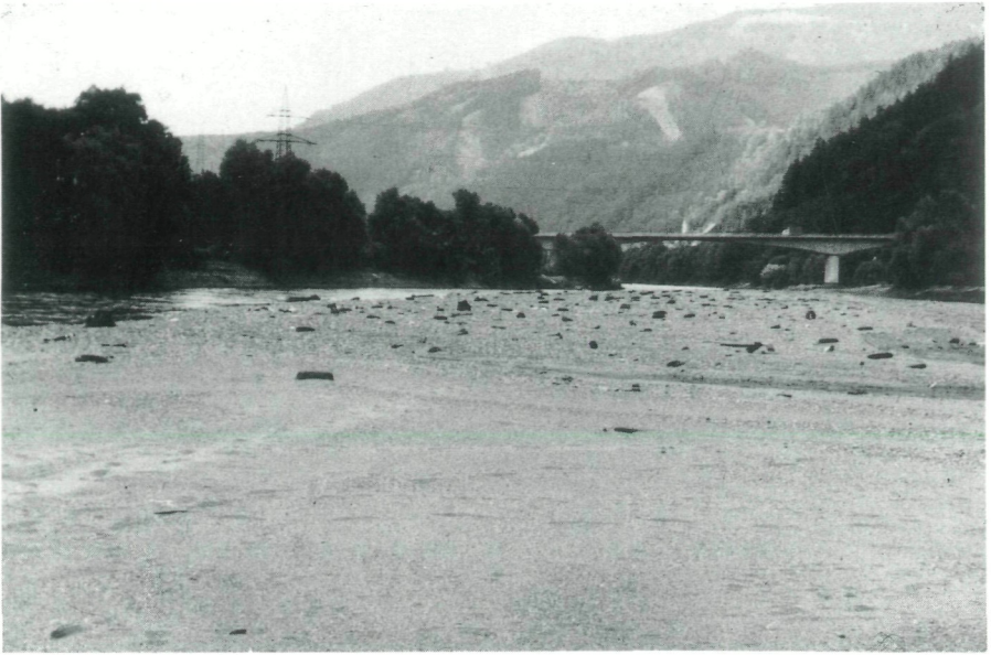
Abb. 1: Der Stauraum Pernegg im abgelassenen Zustand. Beachte die Müllschicht im Bereich der longitudinalen Kiesbarre.
