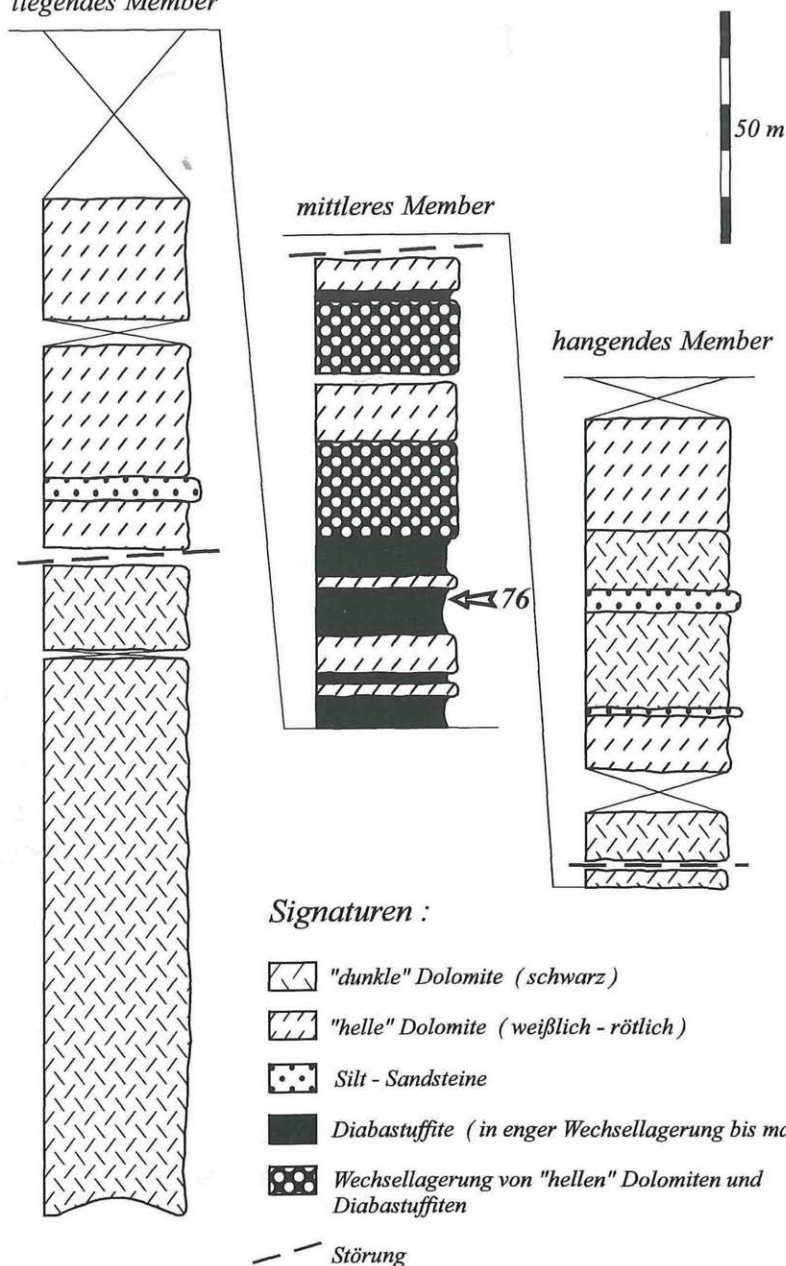
Abb. 1: Profil durch die Dolomitsandstein Formation entlang des Forstaufschließungsweges am Westhang des Admonterkogel-Kanzelkogelzuges, nördlich von Graz. (ÖK 164 Graz, Profilerstreckung: 47°6'54"N/15°23'35"E. Gr. bis 47°6'58"N/15°22'51"E Gr.). Section of the Dolomitesandstone Formation along the roadcut on the western slope of the Kanzel- and Admonterhill north of Graz. (Austrian map sheet ÖK 164 Graz, Profile extension: 47°6'54"N/15°23'35"E. Gr. to 47°6'58"N/15°22'51"E Gr.).
