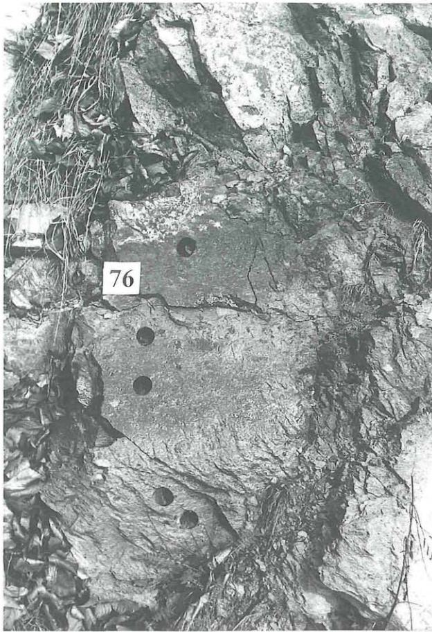
Abb. 2: Tuffitbank, Bildausschnitt 45 cm (Nr. 76; vgl. Abb. 1) Pyroclastic layer, pictorial detail 45 cm (nr. 76; cf. Fig. 1)
