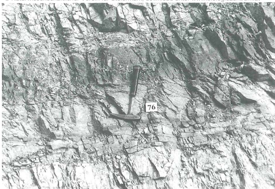
Fig. 1: Aufschlußdetail mit Wechsellagerung von weißen und rosa Dolomiten mit blaugrauen, grauen und violetten Tuffiten. Detail of the investigated outcrop. Alternation of white and pink dolostones with bluish-gray, gray and dusky-red pyroclasts.
