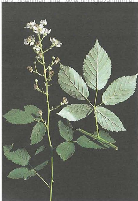
Fig. 31: Rubus montanus LIBERT EX LEJEUNE
