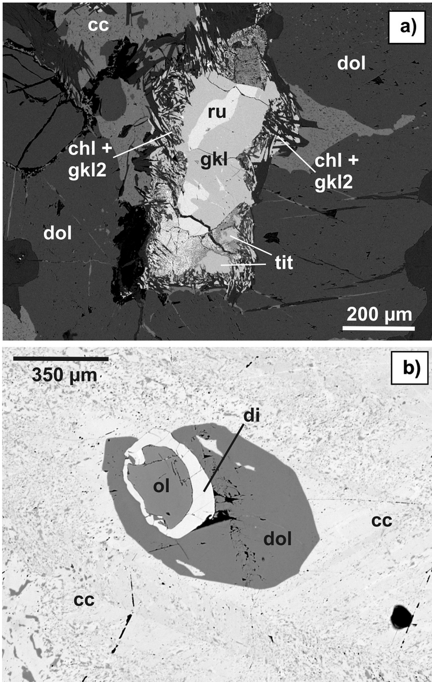
Abb. 2: Rückstreuungselektronen-Bilder von: a) komplexer Verwachsung von Rutil (ru), Geikielith (2 Generationen: gkl1, gkl2) und Titanit (tit) mit Chlorit (chl) in einer Matrix aus Dolomit (dol) und Calcit (cc) (Rhodopengebirge); b) Silikatminerale in Marmor; Backscattered electron images of a) complex intergrowth of rutil (ru), geikielith (2 generations: gkl1, gkl2) and titanite (tit) with chlorite (chl) in a matrix of dolomite (dol) and calcite (cc) (Rhodope); b) silicate minerals in marble;
