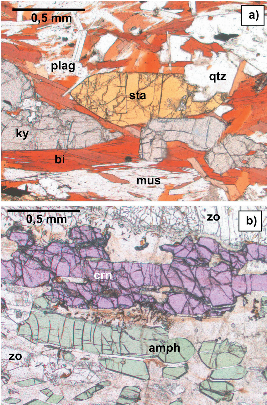
Abb. 1: Mit dem Polarisationsmikroskop gemachte Dünnschliff-Aufnahmen: a) Staurolith (sta), Kyanit (ky) und Biotit (bi) in einer farblosen Matrix von Helleglimmer (mus), Quarz (qtz) und Plagioklas (plag); b) rötlicher Rubin (crn), grüner Amphibole (amph), weißer Zoisit (zo) und feinkörniger brauner Cr-Spinell in einer sehr feinkörnigen mattweißen Matrix (zumeist Margarit); Longido, Tansania; Polarised light microphotographs of a) staurolite (sta), kyanite (ky) and biotite (bi) in a colorless matrix of muscovite (mus), quartz (qtz) and plagioclase (plag); b) pink ruby (crn), green amphibole (amph), white zoisite (zo) and fine-grained brown Cr-spinel in a very fine-grained whitish matrix of mainly margarite; Longido, Tanzania;
