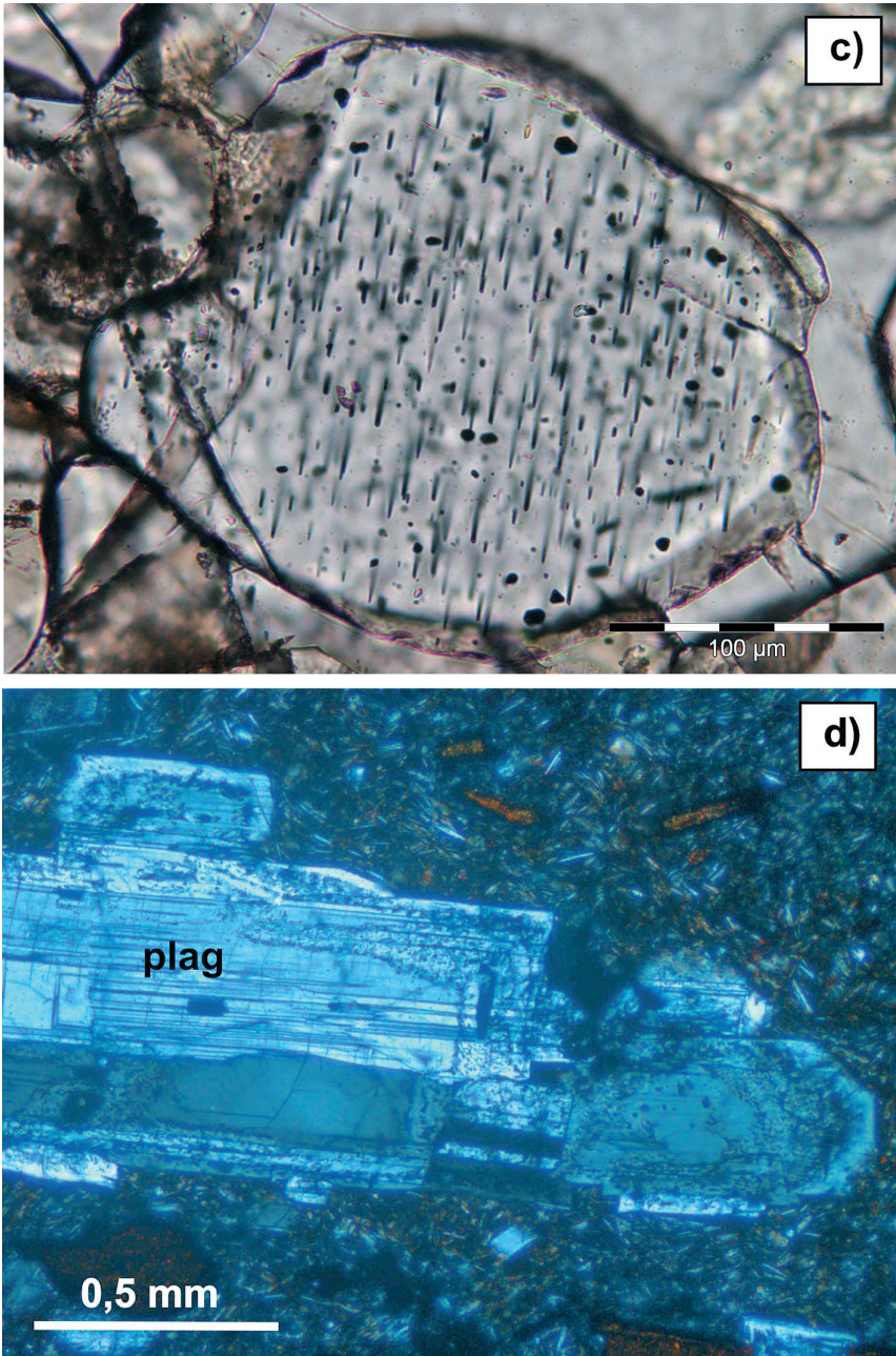
Abb. 1: c) Apatitkristall mit orientierten nadeligen Einschlüssen von Magnetkies (Granulit, Rhodopengebirge); d) zonar gebauter Plagioklaskristall in der feinkörnig entglasten Matrix eines Basaltes (Oststeiermark); Aufnahme mit gekreuzten Polarisatoren. c) apatite crystal with oriented acicular inclusions of pyrrhotite (from a granulite, Rhodope); d) zoned plagioclase crystal in a fine-grained devitrified matrix of a basalt (Eastern Styria), crossed polarisers.
