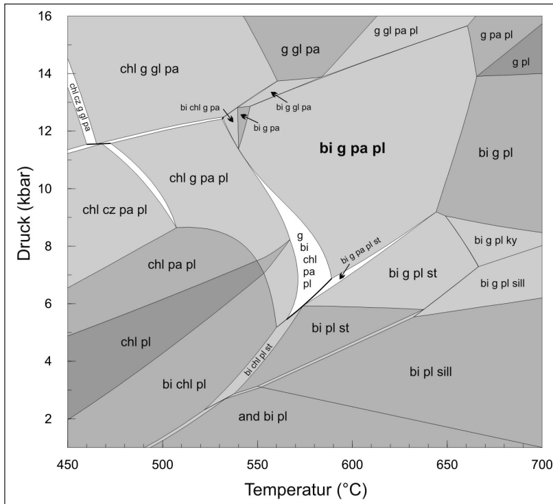
Abb. 3: Pseudoschnitt für einen Glimmerschiefer (Schneebergerzug, Südtirol). Abkürzungen: and = Andalusit, chl = Chlorit, cz = Klinkzoisit, g = Granat, gl = Glaukophan, ky = Kyanit, pa = Paragonit, pl = Plagioklas, st = Staurolith.
