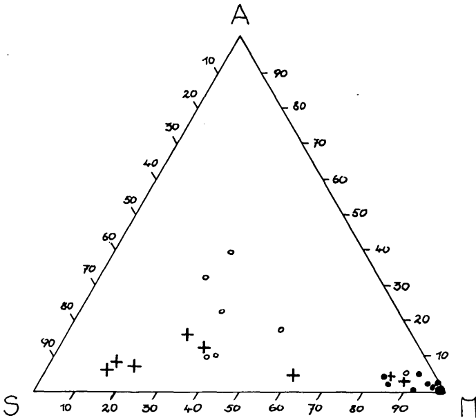
Abb. 3: Darstellung der untersuchten Proben im Mikrit (M) — Sparit (S) — Komponenten (A) Dreieck. Zeichen: + Klobenwandkalk i. e. S., o Lanaukalk, • Scheiblingkalk.
