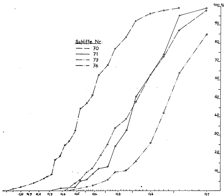
Abb. 2: Korngrößen-Summenlinie (Schliff-Ausmessung) der Intraklaste des Lanauskalkes, Ordinate: \phi in mm. (Gez. auf Din. 8124 T log Modul 160).
