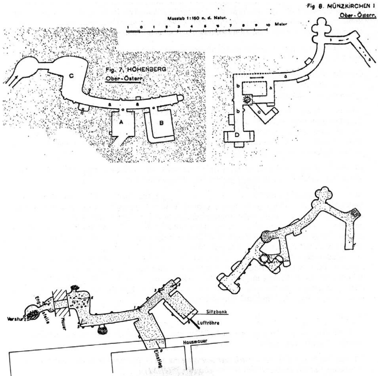
Planvergleich Oben 2 Vermessungspläne von P. Karner Unten die gleichen Anlagen in neuer Aufnahmetechnik
