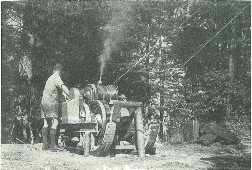
Abb. 1. Das Gerät beim Aufseilen von Lä- und Fi-Blöchen zur Lainaustraße Zug- und Rückholseil laufen über Umlenkrollen, die auf einer Buche oberhalb des Weges verankert sind.
