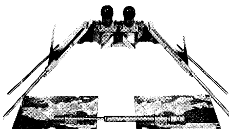
Spiegelstereoskop Wild ST4 mit Binokularaufsatz und Stereomikrometer
