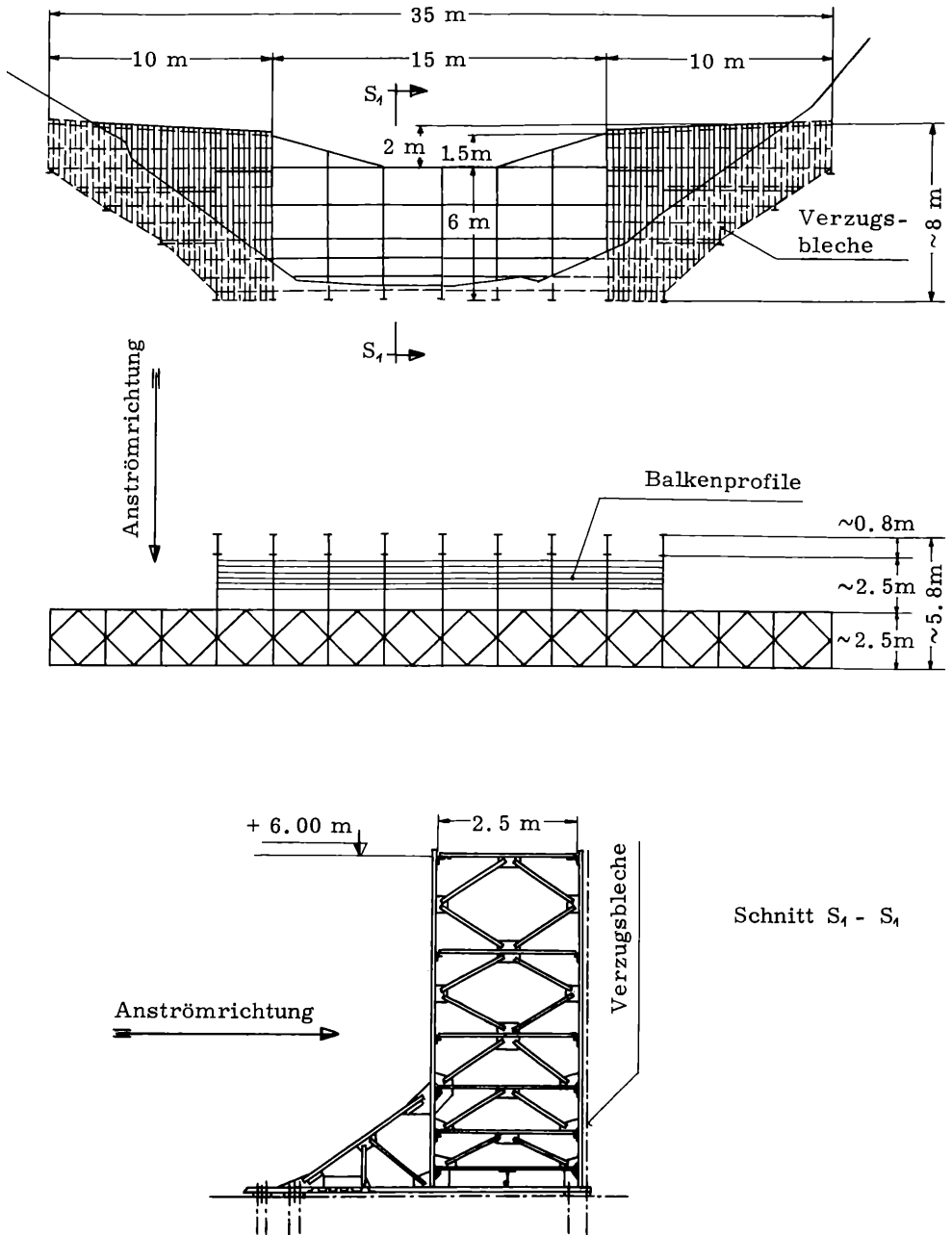
Abb. 22: Konstruktion der Gitterrostsperre im Dürnbach
