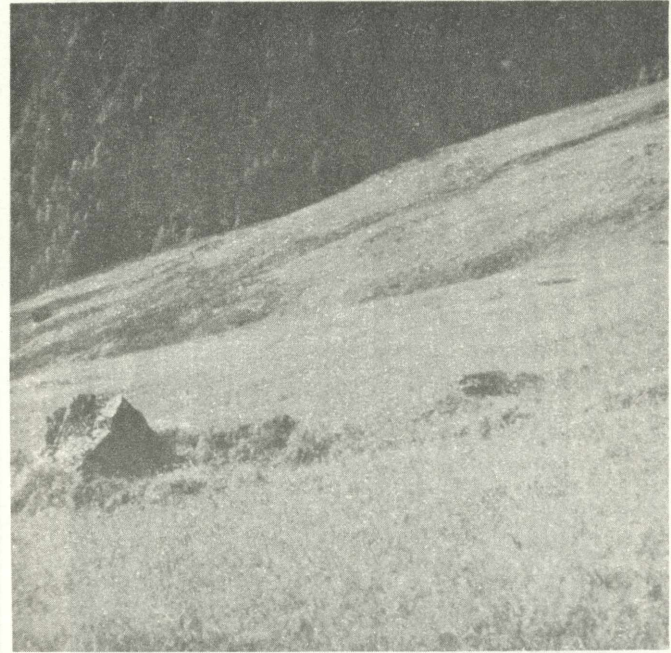
Abb. 4: Solifluktionerscheinungen am Oberhang des Haggener Sonnbergs: Große Steine, die langsam talwärts gleiten, haben einen Erdwulst vor sich aufgeschoben.
