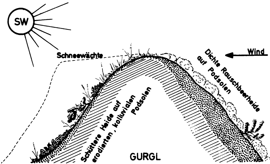
Abb. 7: Skizze des Einflusses von Wind und Schnee auf die Bodenbildung am Haggener Sonnberg und in der Gurgler Heide, Ötztal
