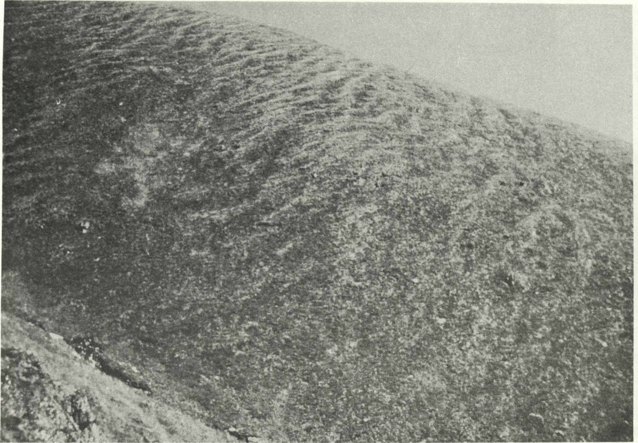
Abb. 3: Solifluktionserscheinungen am Oberhang des Haggener Sonnbergs: Girlandenbildungen der Podsole in SW-Exposition
