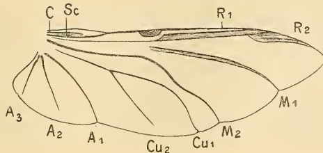
Fig. 3. Hinterflügel von Necrophorus vespilloides Herbst nach Kempers.
