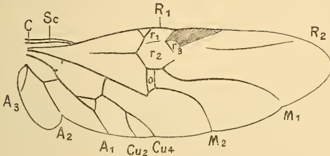
Fig. 2. Hinterflügel von Tachypus flavipes L. nach Kempers.
