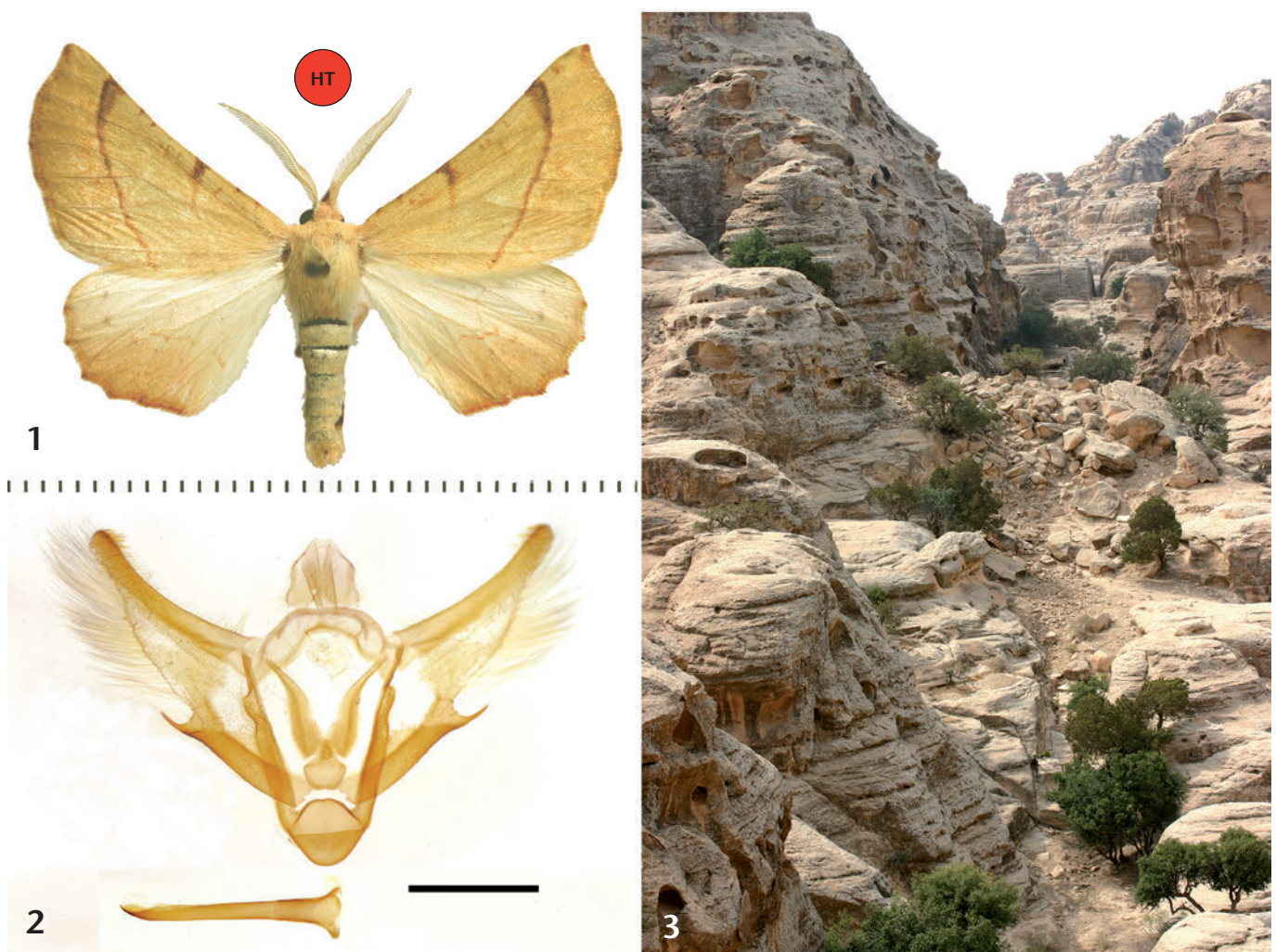
Abb. 1: Eumera lewandowskii sp. nov. Holotypus ♂, Jordanien, Provinz Aqaba, Wādī Mūsá, 9. x. 2007, 1030 m, leg. LEWANDOWSKI & TOBER, coll. LEWANDOWSKI (CSLM), später ZSM. Maßstab in mm. Abb. 2: Eumera lewandowskii sp. nov., männliche Genitalarmatur, GP SL 89, Maßstab ca. 1 mm. Abb. 3: Falterhabitat in Südwestjordanien. – Alle Fotos S. LEWANDOWSKI.
