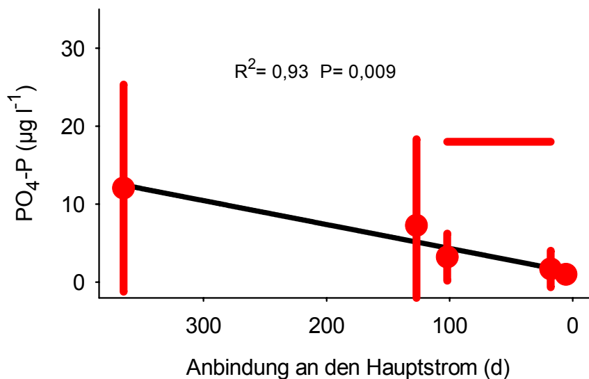
Abb. 6: Abhängigkeit der Orthophosphatkonzentrationen (MW±STABW) von der Anbindungsdauer an die Donau (Einfluss rückstauender Hochwässer). Der rote Balken markiert den Maßnahmenbereich. Die Regression bezieht sich auf die Mittelwerte.
