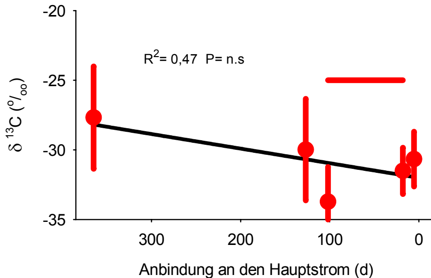
Abb. 5: Abhängigkeit der \delta^{13}\text{C} Werte (MW \pm STABW) von der Anbindungsdauer an die Donau (Einfluss rückstauer Hochwässer). Der rote Balken markiert den Maßnahmenbereich. Die Regression bezieht sich auf die Mittelwerte.
