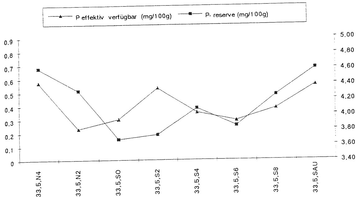
Abb.26: Darstellung des effektiv verfügbaren Phosphors (linke Achse) sowie des Reservephosphors (rechte Achse) in mg/100g nach der EUF-Methode bei Km 33,5.
