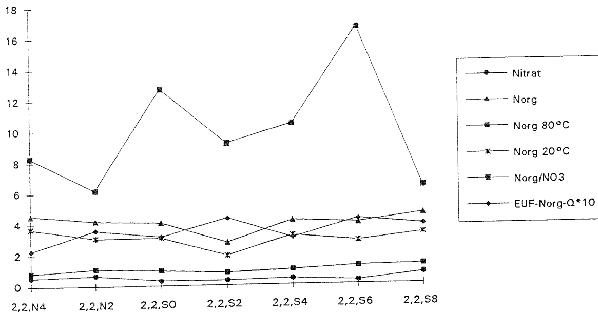
Abb.19: Darstellung des Nitratstickstoffes und des leicht hydrolysierbaren organischen Stickstoffes (Norg.) in mg/100g (davon der mobilere Anteil (Norg 20°C), der standortspezifische Anteil (Norg 80°C)) sowie das Verhältnis von organischem zu anorganischem Stickstoff und das Zehnfache des EUF-Norg-Q bei Km 2,2.
