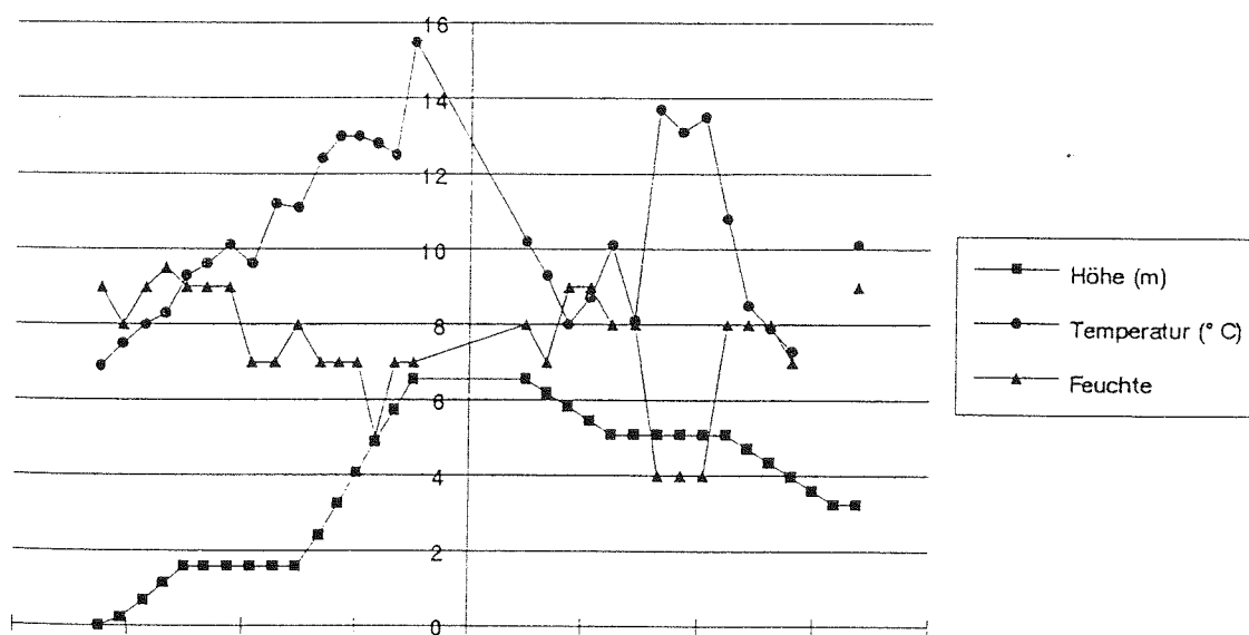
Abb.3: Temperatur-Feuchte-Profil, km 20,5 vom 14.4.1993 14h 30 bei Sonnenschein.
