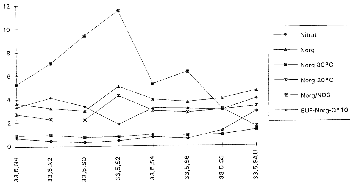
Abb.21: Darstellung des Nitratstickstoffes und des leicht hydrolysierbaren organischen Stickstoffes (Norg.) in mg/100g (davon der mobilere Anteil (Norg 20°C), der standortspezifische Anteil (Norg 80°C)) sowie das Verhältnis von organischem zu anorganischem Stickstoff und das Zehnfache des EUF-Norg-Q bei Km 33,5.
