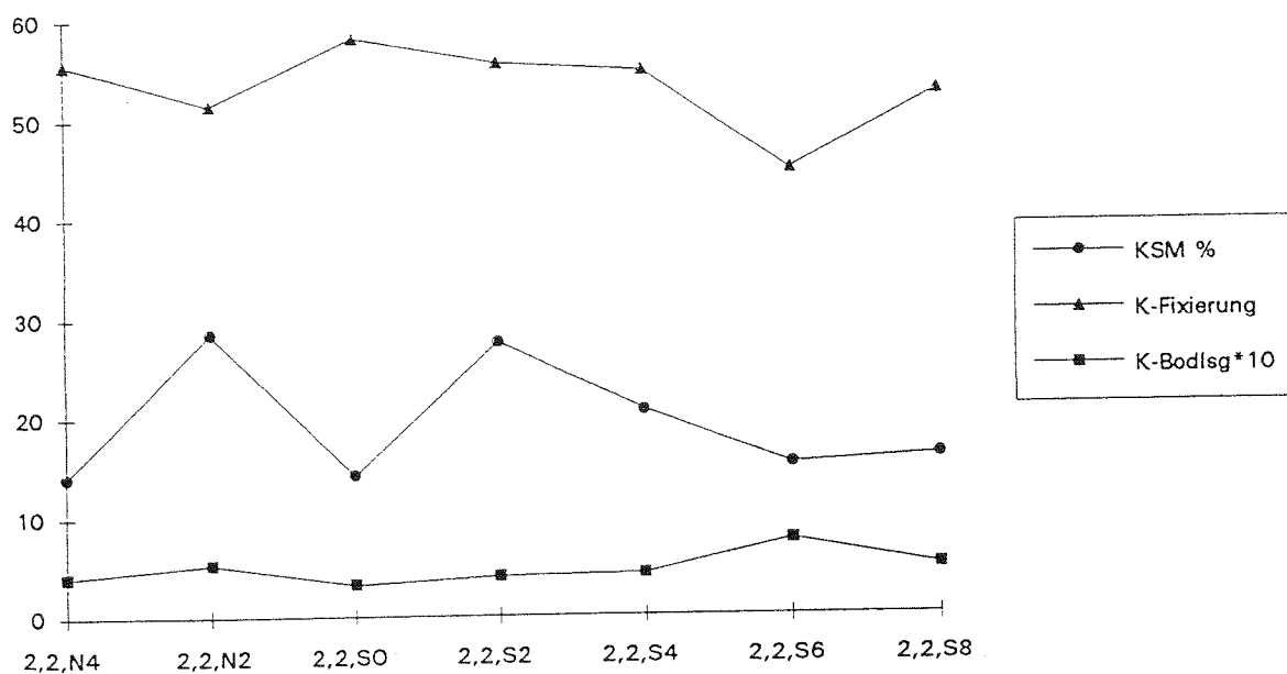
Abb.14: Darstellung des Anteils Kaliumselektiver Minerale in % (KSM), der möglichen Kaliumfixierung in mg/100g und des Zehnfachen der Kaliumkonzentration in der Bodenlösung in mval/l bei Km 2,2.
