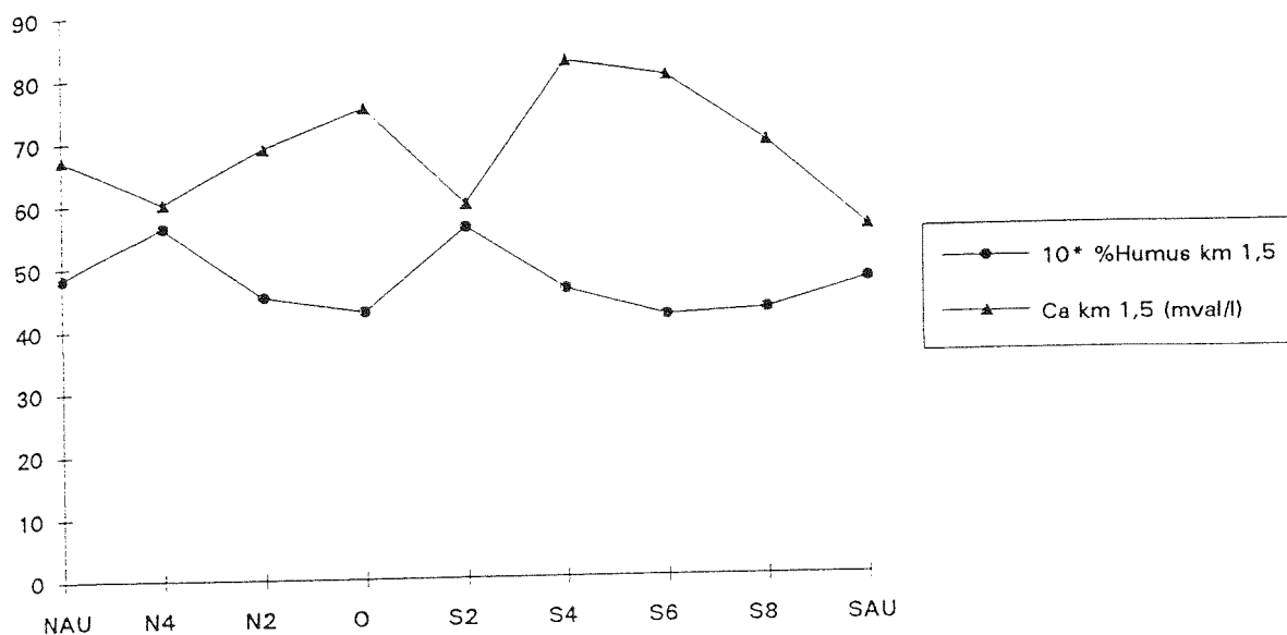
Abb.10: Graphische Darstellung der Ca-Konzentrationen der Bodenlösung (mval/l) im Vergleich zum Gehalt an oxydierbarer Substanz (Humusbestimmung) (10* % oxydierbare Substanz) bei Km 1,5.
