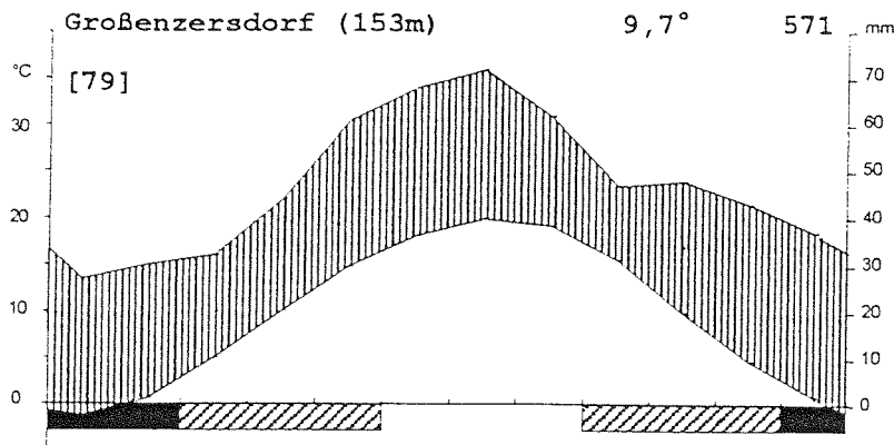
Abb.1: Klimadiagramm von Großenzersdorf erstellt aufgrund der Daten in BEITRÄGE ZUR HYDROGRAPHIE ÖSTERREICHS 1983.
