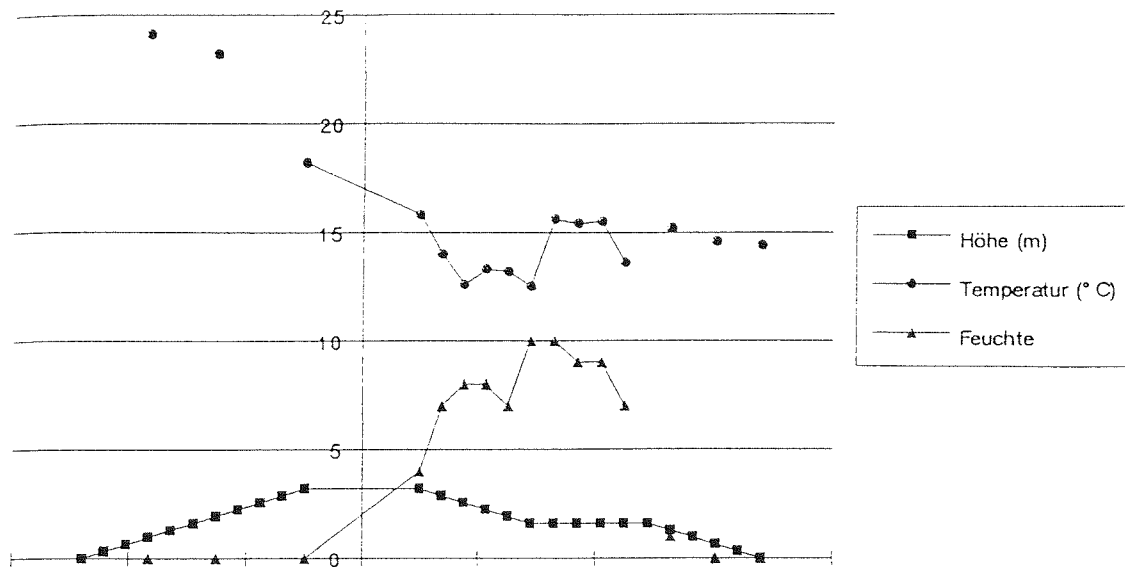
Abb.4: Temperatur-Feuchte-Profil, km 45,5 vom 22.4.1993 13h 30 bei Sonnenschein und starkem Südwind.
