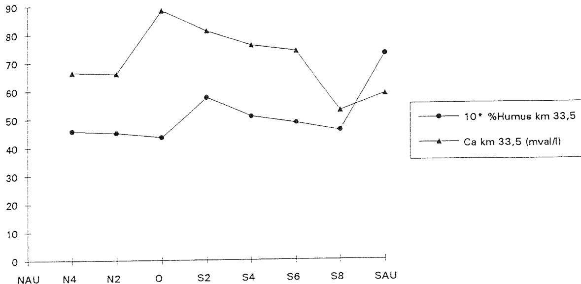
Abb.12: Graphische Darstellung der Ca-Konzentrationen der Bodenlösung (mval/l) im Vergleich zum Gehalt an oxydierbarer Substanz (Humusbestimmung) ( 10 \cdot \% \text{ oxydierbare Substanz} ) bei Km 33,5.
