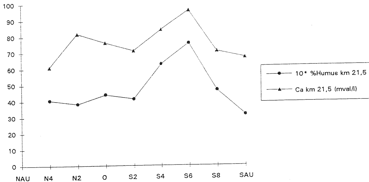
Abb.11: Graphische Darstellung der Ca-Konzentrationen der Bodenlösung (mval/l) im Vergleich zum Gehalt an oxydierbarer Substanz (Humusbestimmung) (10* % oxydierbare Substanz) bei Km 21,5.
