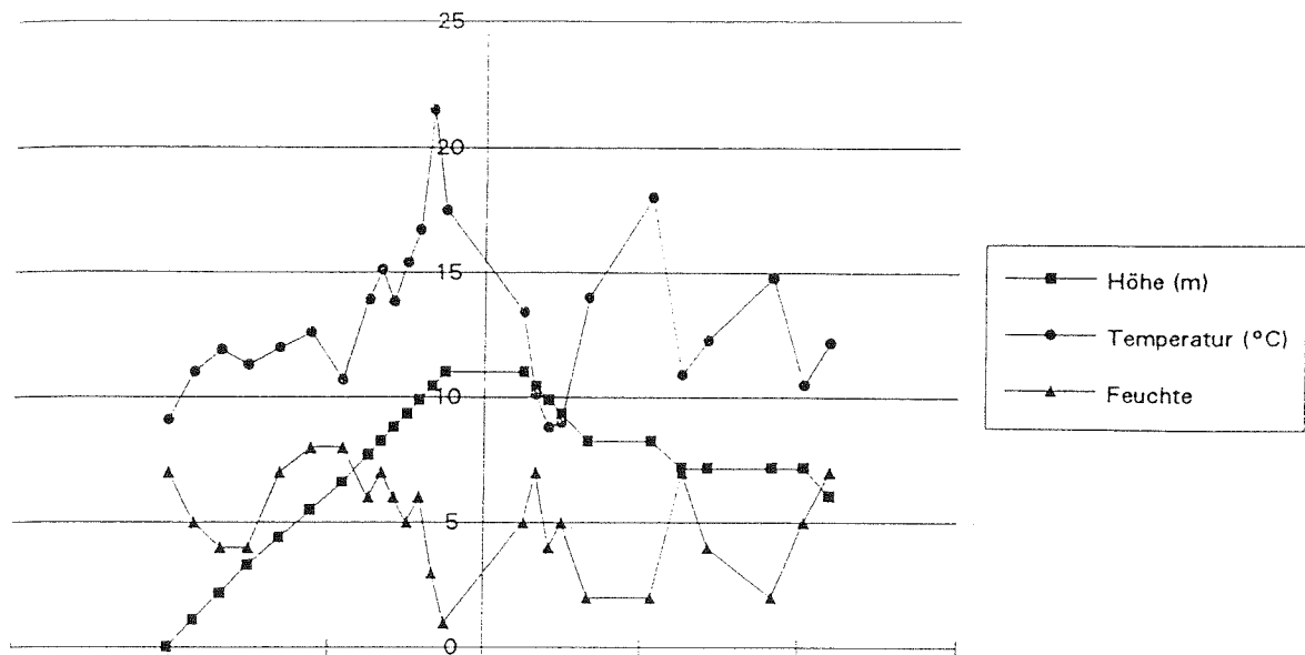
Abb.6: Temperatur-Feuchte-Profil, km 34,5 vom 31.3.1994 bei Sonnenschein und 21°C Lufttemperatur.
