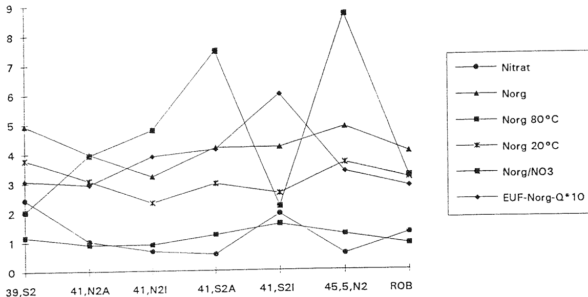
Abb.22: Darstellung des Nitratstickstoffes und des leicht hydrolysierbaren organischen Stickstoffes (Norg.) in mg/100g (davon der mobilere Anteil (Norg 20°C), der standortspezifische Anteil (Norg 80°C)) sowie das Verhältnis von organischem zu anorganischem Stickstoff und das Zehnfache des EUF-Norg-Q bei weiteren Probestellen.
