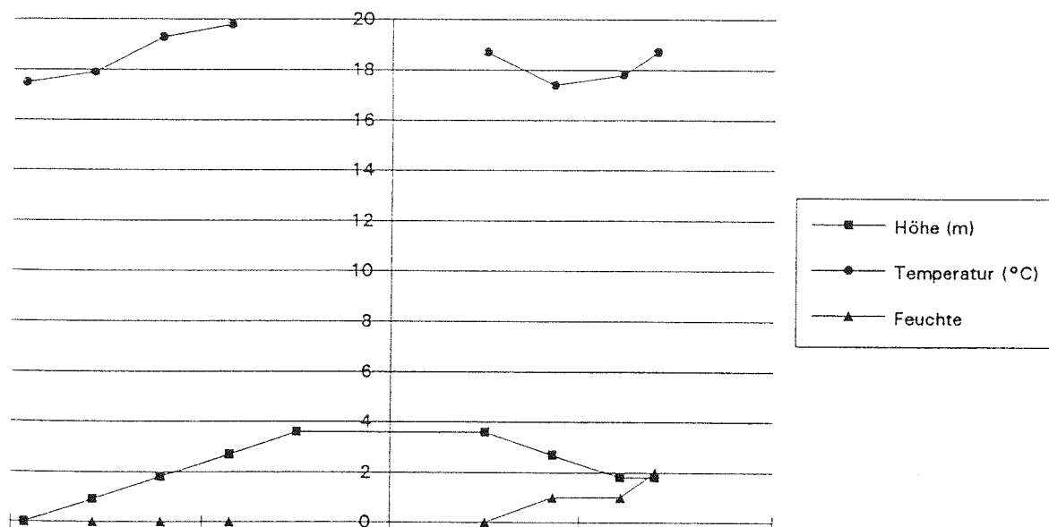
Abb.7: Temperatur-Feuchte-Profil, km 2,4 vom 26.5.1993 14h.
