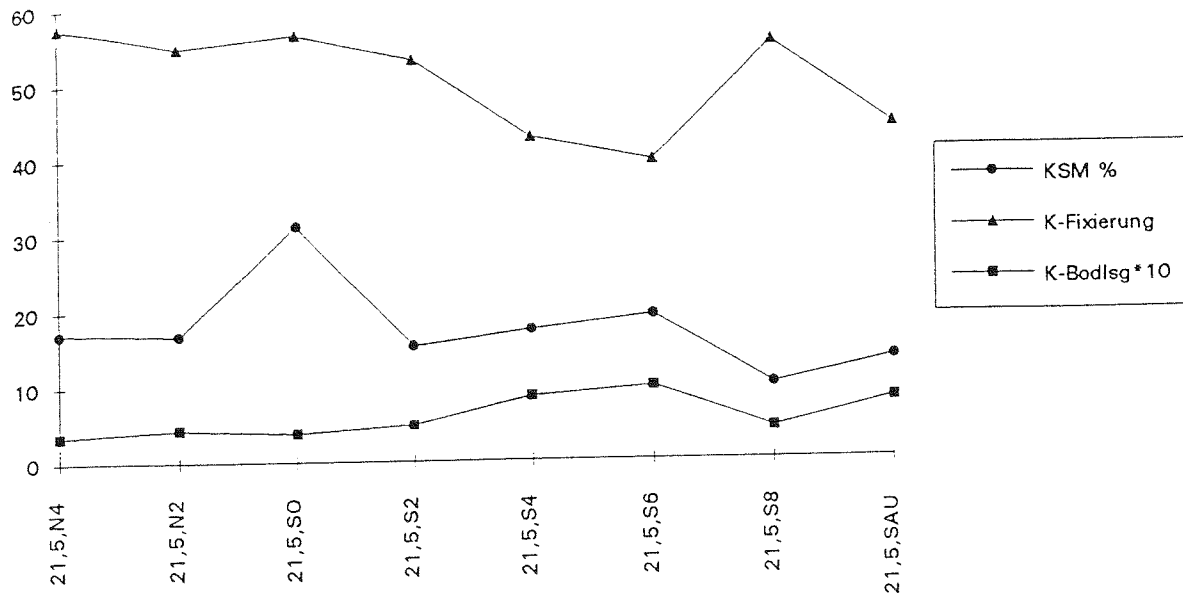
Abb.15: Darstellung des Anteils Kaliumselektiver Minerale in % (KSM), der möglichen Kaliumfixierung in mg/100g und des Zehnfachen der Kaliumkonzentration in der Bodenlösung in mval/l bei Km 21,5.
