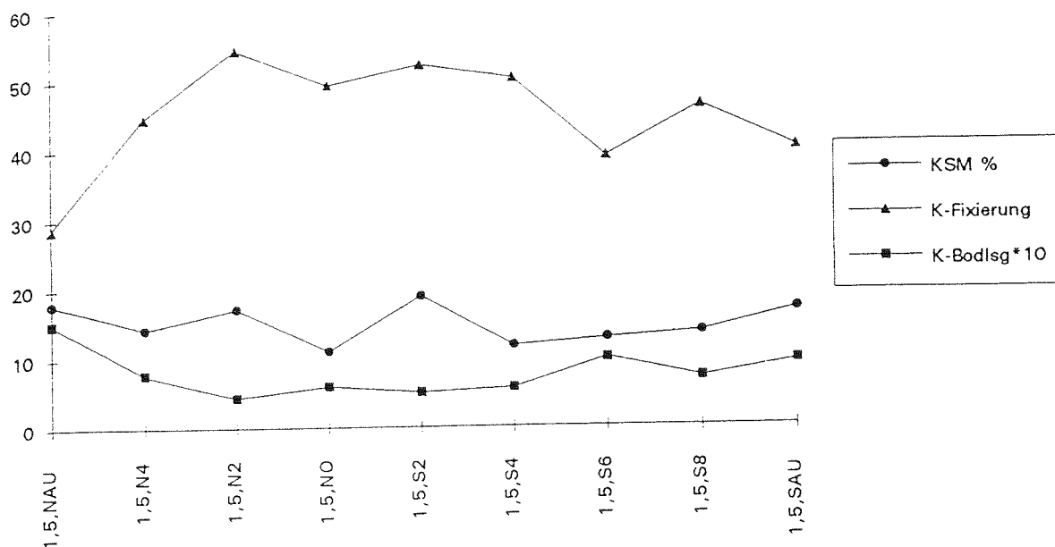
Abb.13: Darstellung des Anteils Kaliumselektiver Minerale in % (KSM), der möglichen Kaliumfixierung in mg/100g und des Zehnfachen der Kaliumkonzentration in der Bodenlösung in mval/l bei Km 1,5.
