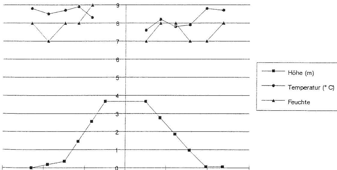
Abb.5: Temperatur-Feuchte-Profil, km 16,5 vom 16.5.1994 14h bei mäßiger Bewölkung und einer Lufttemperatur 14,5 °C.
