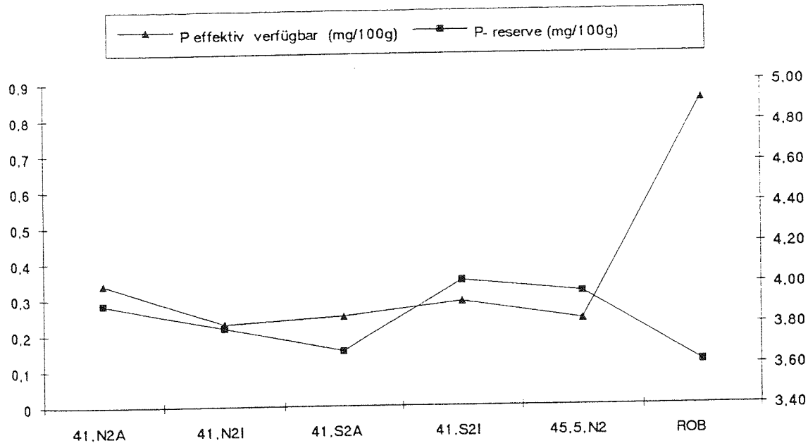
Abb.27: Darstellung des effektiv verfügbaren Phosphors (linke Achse) sowie des Reservephosphors (rechte Achse) in mg/100g nach der EUF-Methode bei weiteren Meßstellen.
