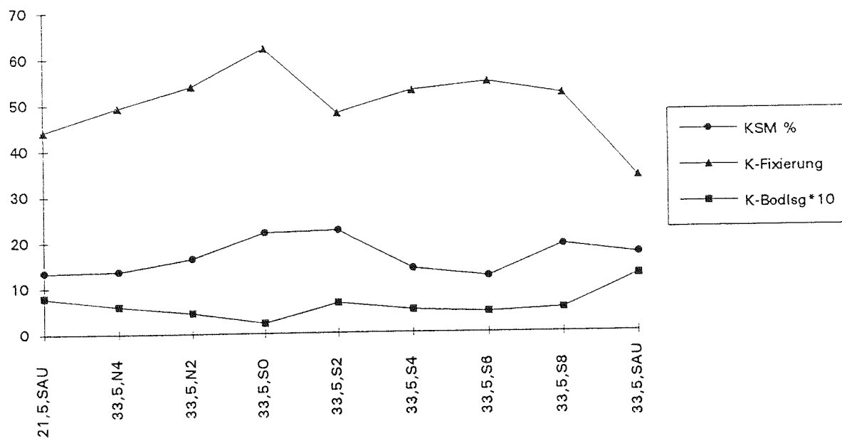
Abb.16: Darstellung des Anteils Kaliumselektiver Minerale in % (KSM), der möglichen Kaliumfixierung in mg/100g und des Zehnfachen der Kaliumkonzentration in der Bodenlösung in mval/l bei Km 33,5.
