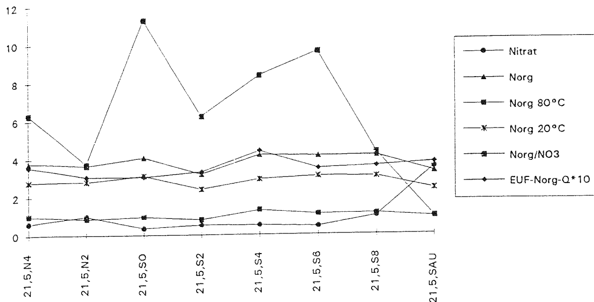
Abb.20: Darstellung des Nitratstickstoffes und des leicht hydrolysierbaren organischen Stickstoffes (Norg.) in mg/100g (davon der mobilere Anteil (Norg 20°C), der standortspezifische Anteil (Norg 80°C)) sowie das Verhältnis von organischem zu anorganischem Stickstoff und das Zehnfache des EUF-Norg-Q bei Km 21,5.
