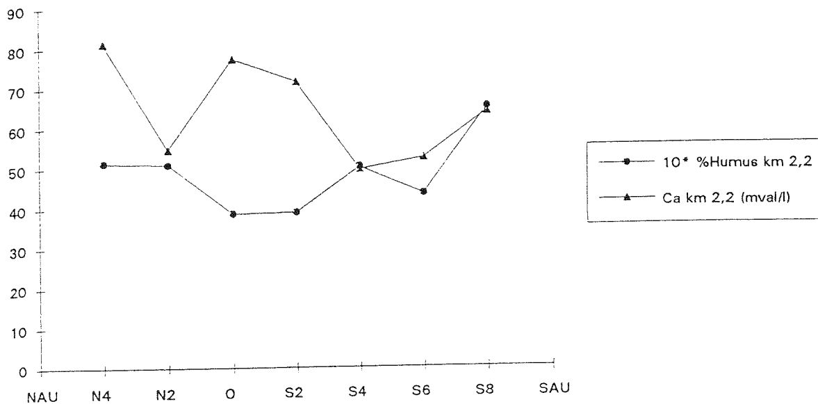
Abb.9: Graphische Darstellung der Ca-Konzentrationen der Bodenlösung (mval/l) im Vergleich zum Gehalt an oxydierbarer Substanz (Humusbestimmung) (10* % oxydierbare Substanz) bei Km 2,2.
