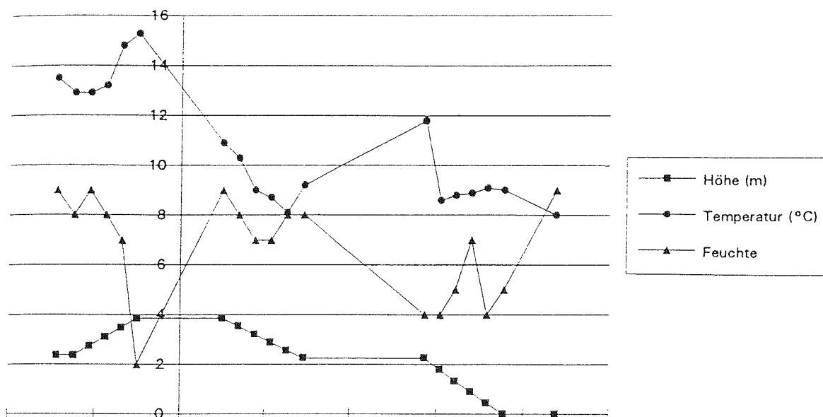
Abb.2: Temperatur-Feuchte-Profil, km 41, vom 17.4.1993 16h 30 bei leichter Bewölkung und mäßigem Wind.
