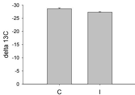
Abb. 7 Delta C13 Werte der Sedimente in den beeinflussten (I) und in den unbeeinflussten Gewässerabschnitten (C) nach Durchführung der Maßnahmen.
