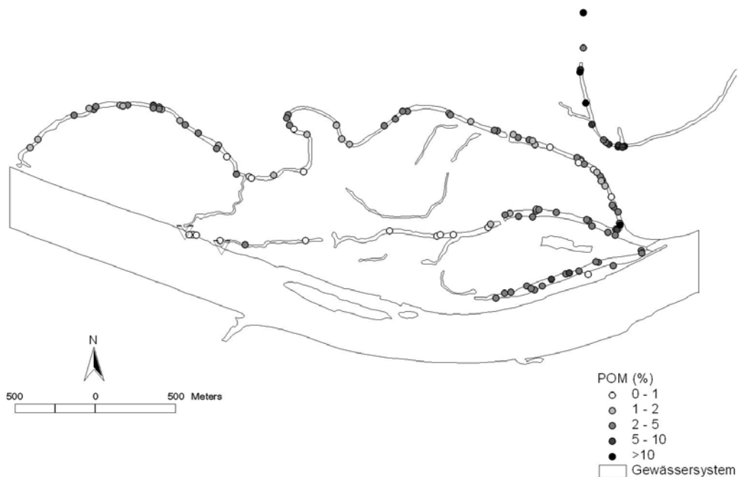
Abb. 5 Räumliche Verteilung des Organischen Gehaltes im Sediment.
