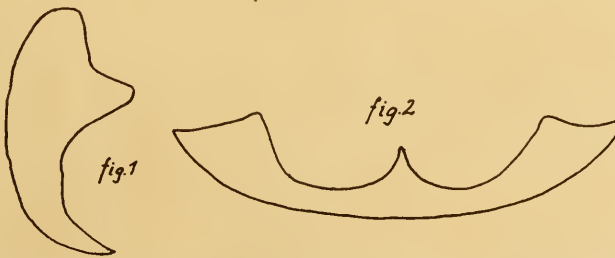
Coniopteryx loipetsederi nov. spec. Hypandrium (schematisiert). Fig. 1: lateral, Fig. 2: ventral.
