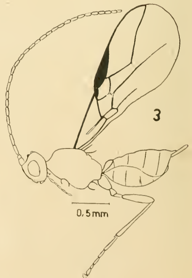
Abb. 2: Opius pallipes Wesmael — Körper in Seitenansicht.
