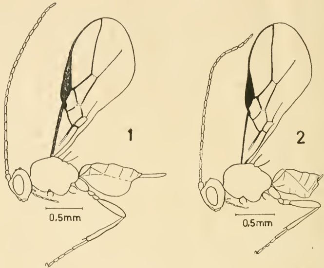
Abb. 1: Opius breviscapus Thomson — Körper in Seitenansicht.
