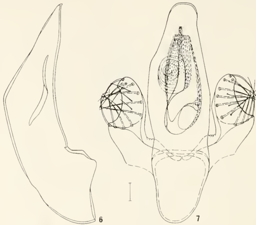
Abb. 6 und 7: Orotrechus jucci POMINI, 1940, vom Locus classicus, Grotta del Mago, Case Vecie, Grezzana, Lessini Veronesi; Aedoeagus Lateral- und Dorsalansicht; Skala 0,10 mm.
