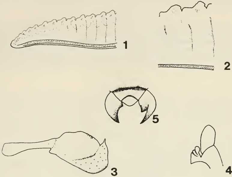
Abb. 2: Linomorpha tricolor MALAISE, -1) Sägevalve, 2) 9.-10. Hauptzahn der Sägevalve, 3) Penisvalve, 4) Parapenis und Harpe, 5) Mundteile.
