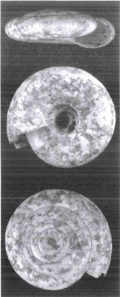
Abb. 1 (links): Balcanodiscus stummerorum nov. spec. von 7 km oberhalb des Klosters Ypapantis to Christo, Pangäon-Gebirge. Abb. 2 (rechts): Der Locus typicus von Balcanodiscus stummerorum nov. spec. 7 km oberhalb des Klosters Ypapantis to Christo, Pangäon-Gebirge.
