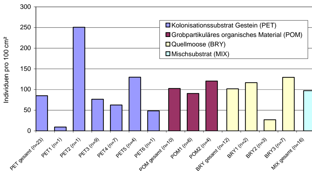
Abb. 27. Individuendichte der Fauna pro 100 cm 2 Gewässerbodenfläche (Probenmittelwert nach semiquantitativer Aufnahme) in den einzelnen Choriotope (Haupt- und Sublebensräume). PET = Gestein (1 = hygropetrische Zone mit epilithischen Algen, 2 = kompaktes Sediment mit epilithischen Algen, 3 = Sedimentumlagerungszone, 4 = lückiges Gewässersediment mit etwas POM-Einlagerung, 5 = Sandbänke, 6 = hydrologisch dynamisch beeinflusste Felsbecken mit dünner Feinsedimentauflage), POM = grobpartikuläres organisches Material (1 = Fallaub jüngerer Datums, 2 = Fallaub jüngerer und älteren Datums mit reichlich Feinmaterial), BRY = Quellmoos (1 = hygropetrischer Charakter, 2 = dichtes Quellmoos in starker Strömung, 3 = Quellmoos mit reichlich eingelagerten Feinmaterial), MIX = Mischsubstrat.
