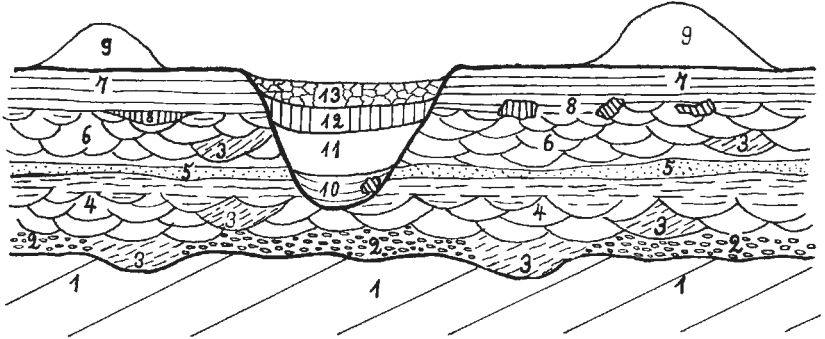
Schematischer Querschnitt durch das Emschertal etwa bei Bottrop-Süd. In der Niederterrasse (1—8) ist eine alluviale Emscherschlinge tief eingegraben und zu- gewachsen (10—13).
