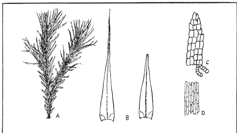
Dicranum strictum Schleich. A) Habitus (4 ×) B) Blätter (10 ×) C) Abgebrochene Blattspitze mit austreibendem Protonema (100 ×) D) Zellnetz der unteren Blathälfte (70 ×)
