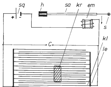
Abb. 1 b. Schaltplan für den Stromkreis C. C = Anschluß des Stromkreises C, em = Elektromagnet, h = Schreibarmhalterung, kl = Kontaktlamelle, kr = Kontakttring am Fuß des markierten Vogels, le = Leitelement aus Lötzinn, s = Registrierschreiber, sa = Schreibarm aus Federmetall, sq = Stromquelle.
