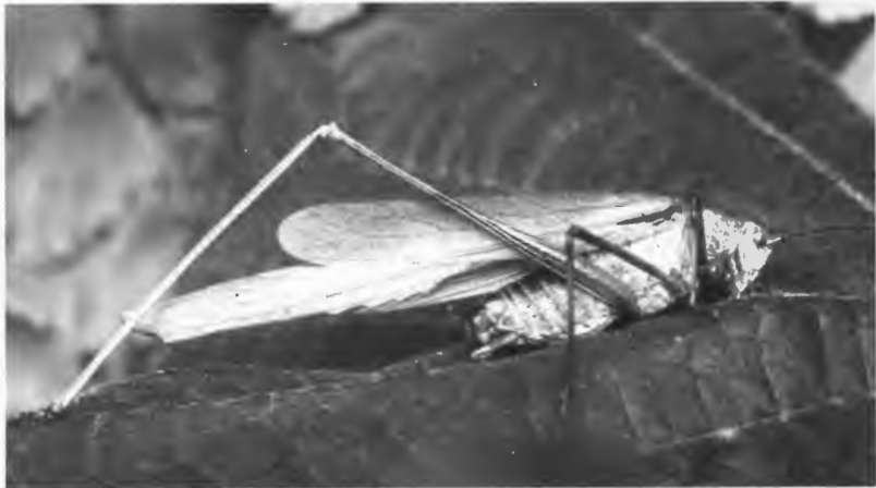
Abb. 2: Phaneroptera falcata -Männchen, Fundort Schwelm/Westfalen
