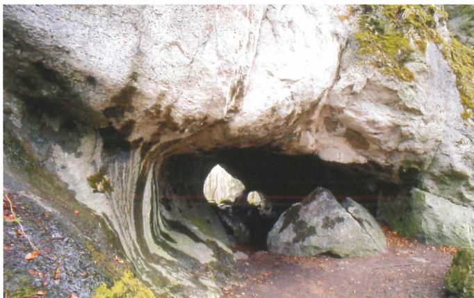
Abb. 24: Der Dolomitfels am „Quackenschloß“ südwestlich Engelhardsberg gibt ein beeindruckendes Beispiel davon, dass auch Brachiopoden wesentlichen Anteil an der Massenfazies des Malm haben können. Die löchrige Felsoberfläche oberhalb des Höhleneingangs ist durch die Herauswitterung tausender Brachiopoden-Steinkerne entstanden. Das Quackenschloß befindet sich allerdings schon im oberen Malm (Malm epsilon), und könnte im Vergleich zum Müllerfels in flacherem Wasser entstanden sein. Foto: Autor.
