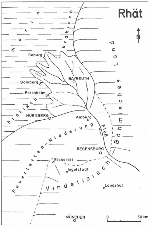
Abb. 17: Der Umbruch des kontinentalen Germanischen Beckens zu einem anhaltend marinen Ablagerungsraum wird östlich Nürnberg dadurch verwischt, dass sich hier die meist grobsandigen Ablagerungen eines von Süden (dem Vindelizischen Land) kommenden Flusses in das Meer vorschieben. Aus MEYER & SCHMIDT-KALER 1992, bzw. BAY. GEOL. LANDESAMT 1996, Erl. GK von Bayern 1 : 500 000, S. 94).
