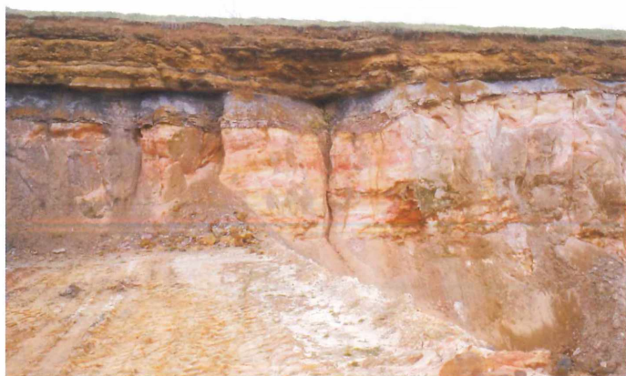
Abb. 19: Noch im Unteren Lias (Lias alpha 3/Arietenschichten) wird schließlich auch das im Rhät angelegte Flussdelta vom Meer überflutet. Die Aufschlusswand zeigt Rhät-Lias-Sandstein, dann eine dunkelgraue Tonsteinlage, darüber die braunen, dünn gebankten Arietenschichten. Letztere sind vorwiegend grobsandig entwickelt und durch ihr sehr eisenreiches, meist karbonatisches Bindemittel relativ abtragungsresistent. Steinbruch östl. Forkendorf (südlich Bayreuth); Foto: Autor.
