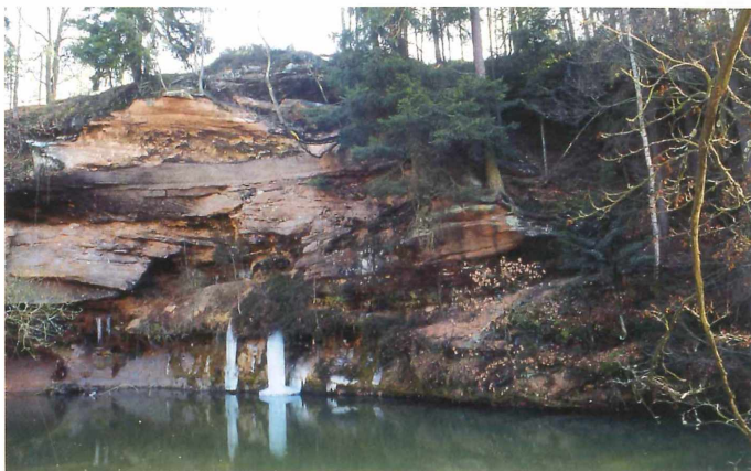
Abb. 9: In der Schwarzachschlucht südlich Nürnberg ist der Burgsandstein vorzüglich erschlossen. Massive Schüttungskörper mit Schrägschichtung sind charakteristische Bildungen von Schwemmfächern im Randbereich des Germanischen Beckens. Foto: Autor.
