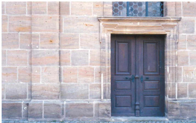
Abb. 14: Bei Lichtenau wird die charakteristische Fazies des Schilfsandsteins durch grobkörnige Schüttungen aus dem südlich gelegenen Vindelizischen Land verdrängt. Der Schilfsandstein (nicht petrografisch, sondern als Formationsbegriff genommen) ist hier kaum von den übrigen grobkörnigen Keupersandsteinen (wie etwa dem Burgsandstein) zu unterscheiden. Grobkörniger Schilfsandstein mit Schrägschichtung, Kirche im alten Ortskern von Lichtenau. Foto: Autor.
