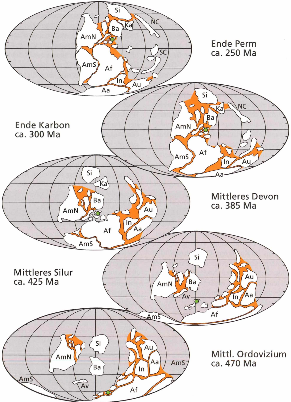
Abb. 3: Die Entstehung des Fundaments von Mitteleuropa im Paläozoikum. Grafiken modifiziert nach Darstellungen von SCOTESE ( www.scotese.com ), der Weg der Mikroplatten zum varistischen Gebirge nach FRANKE et al.2000. Festländische Kontinentalbereiche sind weiß bezeichnet. Die hellbraune Markierung verbindet kontinentale Bereiche, die als plattentektonische Einheit zusammengefasst werden können, wobei eine Bedeckung mit flachen Schelfmeeren möglich war. Abkürzungen: Aa/Antarktis, Af/Afrika, AmN/Nordamerika, AmS/Südamerika, Au/Australien, Av/Avalonia, Ba/Baltischer Schild, In/Indien, Ka/Kasachstan, NC/Nordchina, SC/Südchina, Si/Sibirischer Schild. Die Lage Nürnbergs (grüner Punkt) wäre am Rand oder zwischen zwei Mikroplatten („Saxothuringia“ und „Bohemia“ bzw. „Moldanubia“) anzusiedeln.
