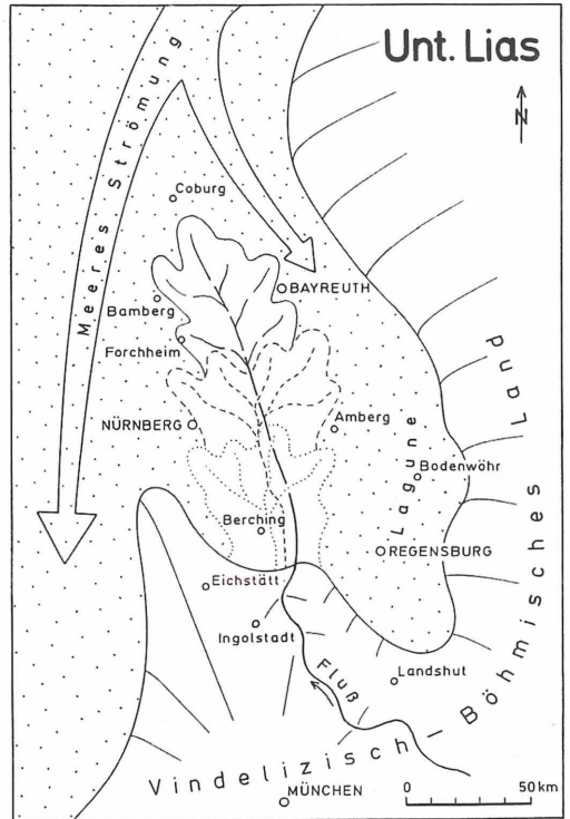
Abb. 17: Der Umbruch des kontinentalen Germanischen Beckens zu einem anhaltend marinen Ablagerungsraum wird östlich Nürnberg dadurch verwischt, dass sich hier die meist grobsandigen Ablagerungen eines von Süden (dem Vindelizischen Land) kommenden Flusses in das Meer vorschieben. Aus MEYER & SCHMIDT-KALER 1992, bzw. BAY. GEOL. LANDESAMT 1996, Erl. GK von Bayern 1 : 500 000, S. 94).
