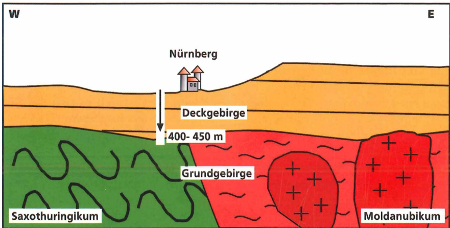
Abb. 2: Schematische Querschnitte zum strukturellen Verhältnis Grund- und Deckgebirge.
