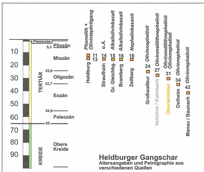
Abb. 3: Tabelle einiger radiometrischer Alter von Vulkaniten der Heldburger Gangschar. Daten nach LIPPOLT in POHL & SOFFEL 1977; HUCKENHOLZ & SCHRÖDER 1981, HUCKENHOLZ & WERNER 1990 sowie nach HAUTMANN et al. in ELLENBERG, SCHRÖDER, PETEREK & MORGENROTH 2001
