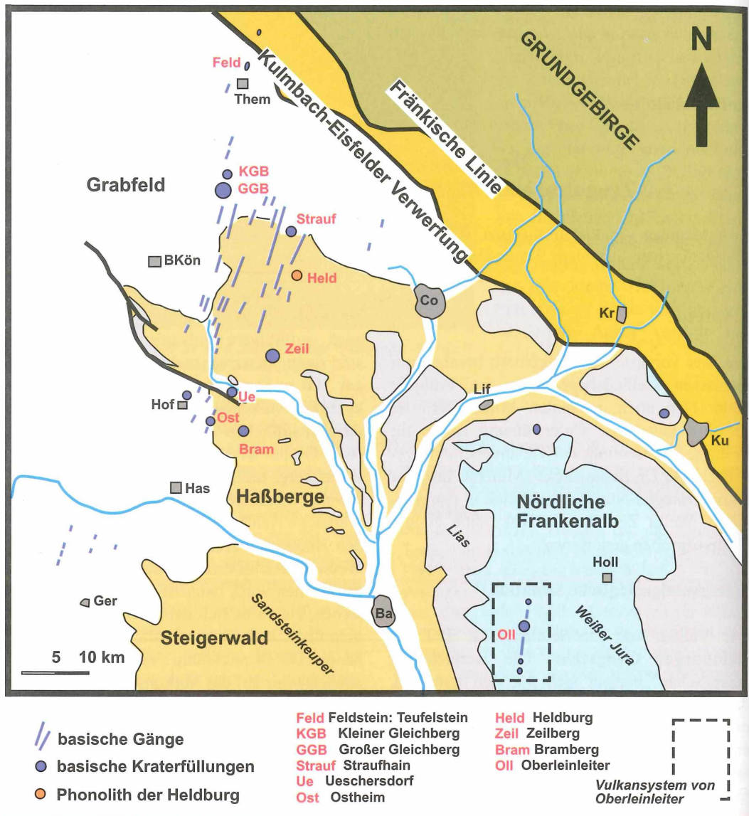
Abb. 1: Geologische Kartenskizze von Nordbayern und Südthüringen, mit Heldburger Gangscharr und Lage des Vulkansystems von Oberleinleiter. Vereinfacht nach Geol. K. Bayern 1:500000 (Bayer. Geol. Landesamt). Ba: Bamberg – BKön: Bad Königshofen – Co: Coburg – Ger: Gerolzhofen – Has: Hassfurt – Hof: Hofheim – Kr: Kronach – Ku: Kulmbach – Lif: Lichtenfels – The: Themar.
