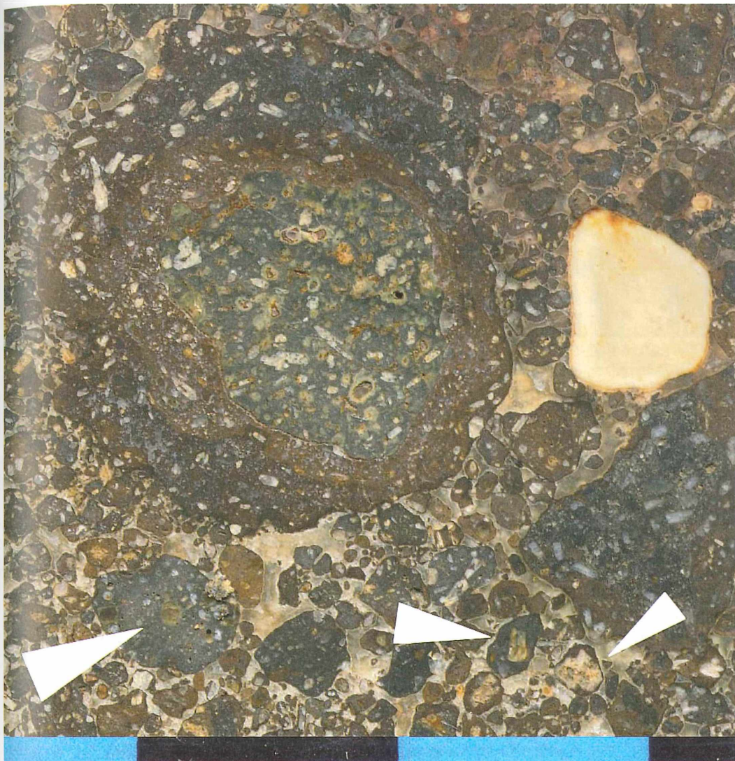
Abb. 10: Lapilli mit Olivinkristallen im Kern (die beiden linken Pfeile), Der rechte Pfeil weist auf einen Lapillus mit Calcit im Kern. In diesen und anderen Fällen sind die Calcite zu groß, als dass sie Blasenfüllungen sein könnten. Vermutlich handelt es sich um Verdrängungseffekte, in erster Linie wohl auf Kosten von Olivin. Der große Lapillus im oberen Bildabschnitt zeigt einen zweiphasigen Aufbau, eine dritte Schale wird durch Verwitterungsfronten vorgetäuscht. Der innere Bereich zeigt zahlreiche stark verwitterte bzw. möglicherweise thermometamorph umgewandelte Einschlüsse. Maßstabs-Einheit: cm.
