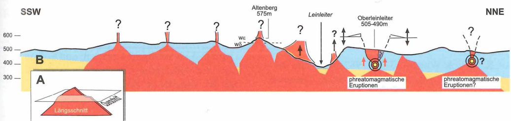
Abb. 15: Idealisiertes modellartiges Längsprofil (B) durch das Vulkansystem von Oberleinleiter. Während ein Gang im Querschnitt nur einen geringen Durchmesser hat (siehe Einlage A), erscheint er im Längsschnitt wie die Wand einer Mauer. Das Modell geht davon aus, dass die einzelnen, an der Oberfläche nachweisbaren vulkanischen Vorkommen Spitzen eines in der Tiefe zusammenhängenden Gangkörpers sind (diese Zusammenhänge sind ohne konkrete empirische Grundlage und daher rein schematisch zu verstehen). Diskussion einzelner Segmente im Text.
