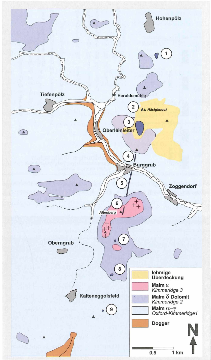
Abb. 2: Geologische Kartenskizze des Vulkansystems von Oberleinleiter, vereinfacht nach Geol. K. Bayern 1:25000, Blätter Buttenheim und Scheßlitz (Bayer. Geol. Landesamt 1972, 1979). Die einzelnen nachgewiesenen vulkanischen Segmente sind von N nach S durchnummeriert.
