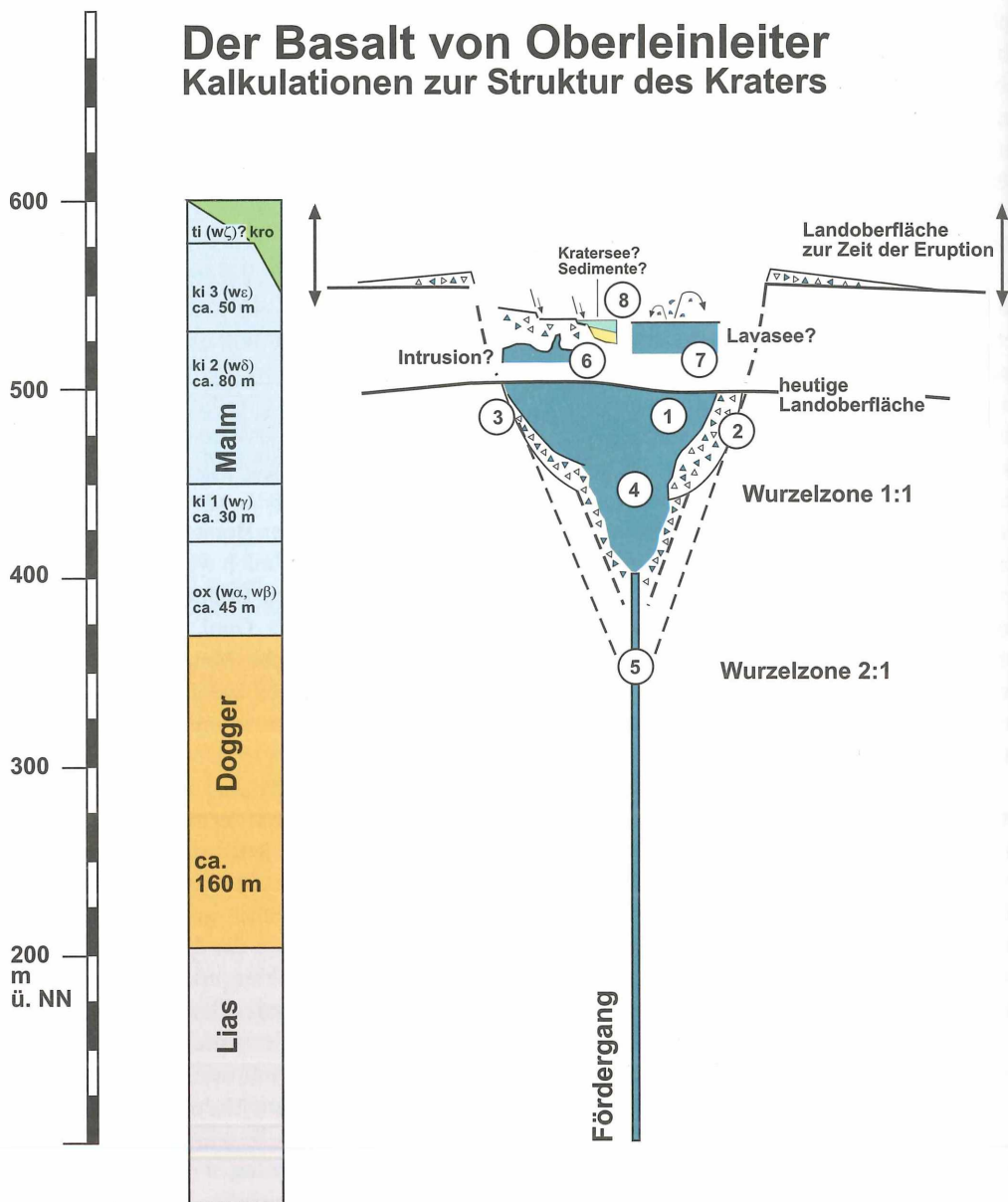
Abb. 12: Modell des Vulkans von Oberleinleiter als ein mit Basalt erfüllter Maarkrater. Die Erklärung der einzelnen Punkte im Text.
