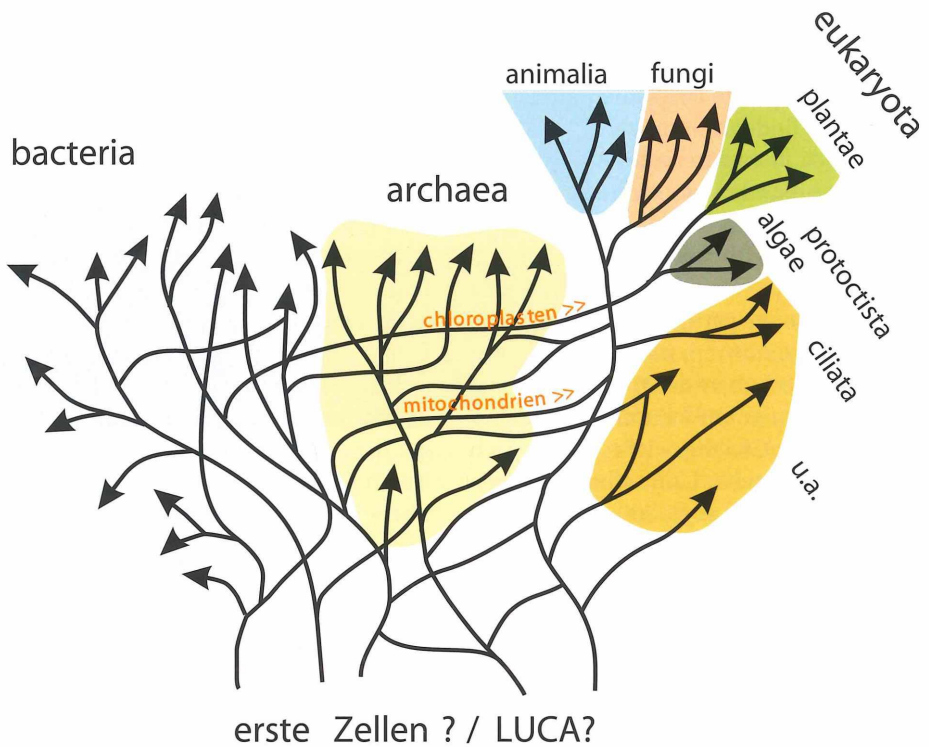
Abb. 6: Der Stammbaum des Lebens unter angemessener Berücksichtigung der Bakterien (in vieler Hinsicht ebenfalls nur schematisch dargestellt). Zwischen den beiden Domänen der Archaea und Bacteria kam es zu erheblichem horizontalem Genaustausch, ohne dass die grundsätzlichen Unterschiede hinsichtlich bestimmter Eiweißformen verwischt wurden. Der horizontale Gentransfer könnte ein Hindernis sein, einen ersten gemeinsamen Vorfahren des Lebens ( Last Universal Common Ancestor, LUCA ) bestimmen zu können. Möglicherweise endet die Suche nach dem ersten Vorfahren bei einem Genpool, den Bakterien durch horizontalen Austausch miteinander geteilt haben. Zellorganellen von Eukaryoten sind durch Symbiose mit aufgenommenen Bakterien entstanden (umgezeichnet nach „v43n2-teske_edwards1en_8591.gif“, woods hole oceanographic institute, http://www.whoi.edu/oceanus/viewImage.do?id=8591&aid=3807 ).
