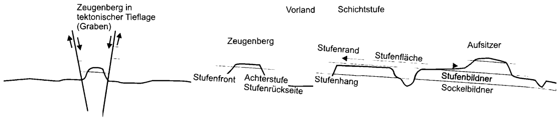
Abb. 1: Schematisches Profil einer Schichtstufen-Landschaft mit einer Verortung der wichtigsten Begriffe
