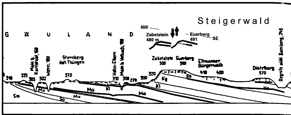
Abb. 2: Ausschnitt aus dem „wahren Profil durch Franken“ (BÜDEL 1957). Die schlechte Abbildungsqualität ist der Vorlage geschuldet. Die von BÜDEL als alte Ebenen/Schnittflächen angesehenen Verebnungen wurden zur besseren Kenntlichkeit gelb hervorgehoben. Rot eingetragen sind Korrekturen zur tektonischen Struktur dieses Ausschnitts. Die Schichtneigung im Bereich der Gäulfläche wurde von BÜDEL zu schematisch dargestellt - in „Wahrheit“ handelt es sich um einen weiten Bereich, der - über die Distanz gesehen - durch eine nahezu ebene oder nur leicht nach Osten gerichtete Lagerung der Schichten gekennzeichnet ist. Die vom Zabelstein zum Euerberg skizzierte Verebnung quert in „Wahrheit“ eine Verwerfung. BÜDEL fasste hier zwei nebeneinander gelegene, durch eine Verwerfung getrennte Stufenfrontbereiche derart zu einem Stufenabschnitt zusammen, dass das Nebeneinander unzutreffenderweise als ein Hintereinander erscheint.
