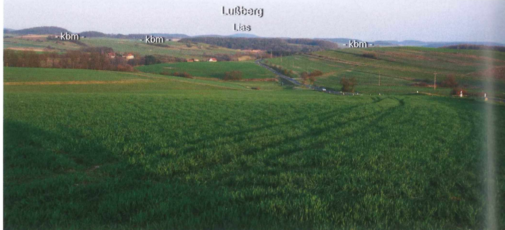
Abb. 17: Im Bereich der südlichen Haßberg-Hochfläche ist - wie auch im Steigerwald - der kbm mit seinen dolomitischen Elementen der morphologisch prägnanteste Stufenbilder. Aufgrund relativ junger tektonischer Verstellungen fällt das Höhenniveau der Stufenfront von 450 m im NW auf ca. 330 m im SE ab. Standpunkt östl. Ortsrand Kottenbrunn, Blick nach SE; die links der Straße im Tal erkennbaren Häuser gehören zur Ortschaft Dörfliß.
