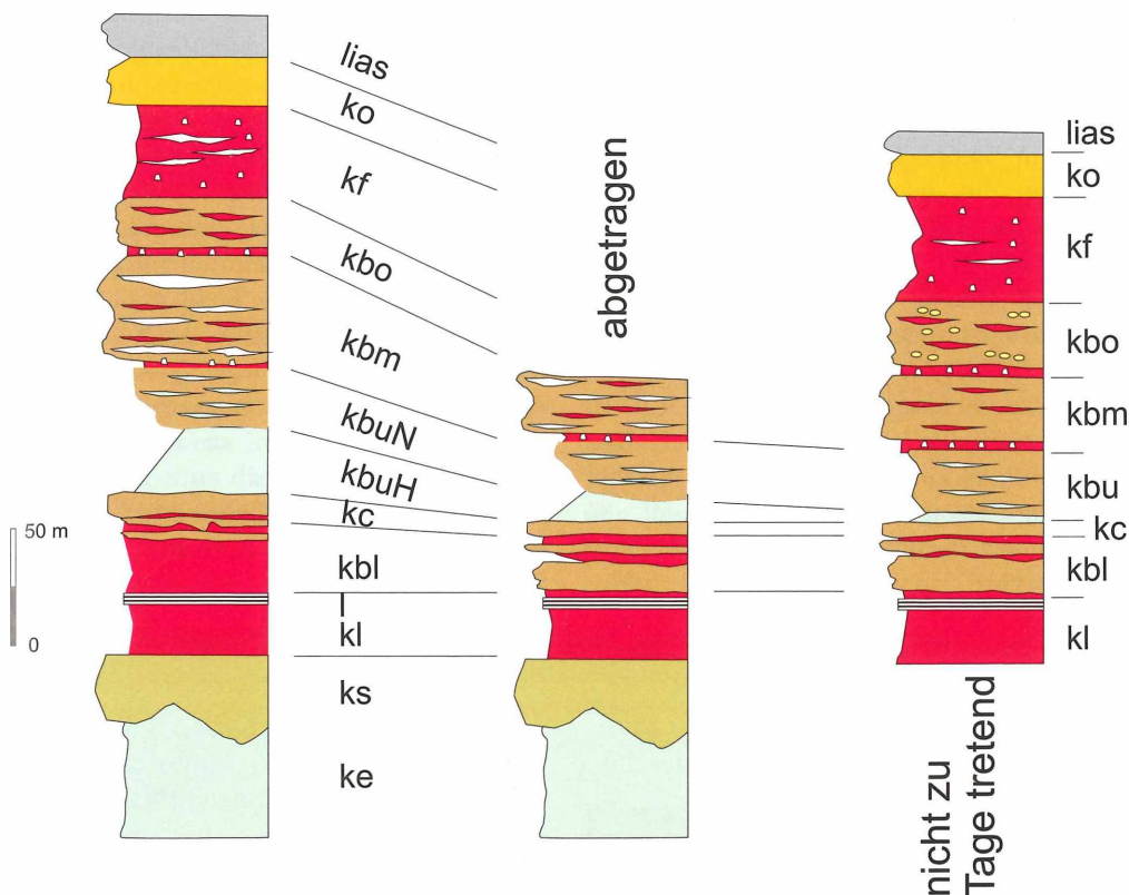
Abb. 4: Schichtenfolge Mittlerer Keuper - Unterer Lias im Steigerwald und den südlichen Haßbergen. - ke Estherienschiefer: Tonsteine, Lehme - ks Schilfsandstein, rinnenartig nach unten in die Estherienschiefer eingreifend - kl Lehrberg-Schichten, oben mit den dolomitischen Lehrberg-Bänken l - kbl Blasensandstein, an der Basis Tone; in den südlichen Haßbergen werden die Sandsteine bis auf die obersten Abschnitte von Tonen und Lehmen verdrängt - kc Coburger Sandstein - kbu Unterer Burgsandstein, zum westlichen Steigerwald hin in eine untere, tonreiche Heldburger Fazies kbuH und eine obere, sandige Nürnberger Fazies kbuN aufspaltend, mit vielfachen linsenartigen Einschaltungen von Zwischenletten - kbm Mittlerer Burgsandstein, zum westlichen Steigerwald und noch mehr zu den Haßbergen hin an Mächtigkeit zunehmend; in dieser Richtung nehmen weiter auch Feldspatgehalt, dolomitische Zementierung und eingelagerte Dolomitbänke zu, so dass von Dolomitischer Arkose gesprochen wird - kbo Oberer Burgsandstein - kf Feuerletten, mit dolomitischen Einlagerungen - ko Oberer Keuper mit Rhätsandstein - lias unterster Lias mit marin gebildetem Angulatussandstein. Die gewählten Kürzel sind an die in den Geologischen Karten 1:25000 üblichen Zeichen angelehnt.
