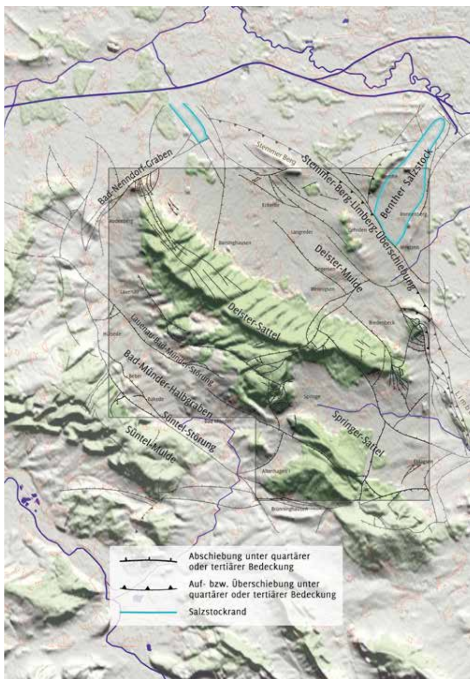
Abb. 1 Geologische Strukturen im Untergrund von Deister und Umland. Der eingrahmte Bereich entspricht der Geologischen Wanderkarte 1:25 000.
