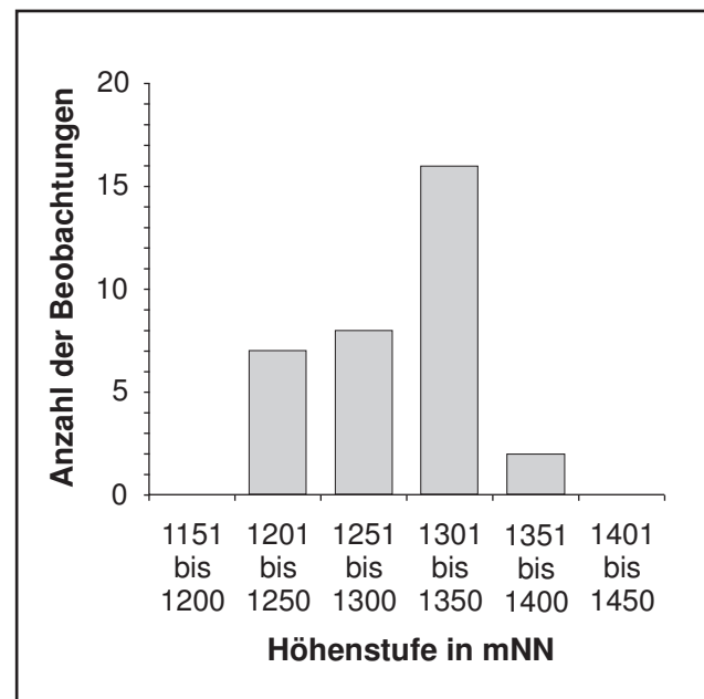
Abb. 2: Die Höhenverbreitung von 33 Nachweisen des Dreizehenspechtes 1982 bis 1994.
