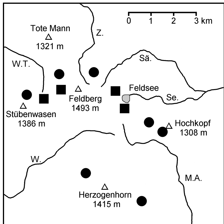
Abb. 1: Vorkommen des Dreizehenspechts im Feldberggebiet. Quadrate : Gebiete mit Brutnachweisen. Kreise : Weitere Gebiete mit Beobachtungen. Abkürzungen : W. : Wiese; W.T. : St. Wilhelmer Talbach; Z. : Zastlerbach; Sä. : Sägebach; Se. : Seebach; M.A. : Menzenschwander Alb.
