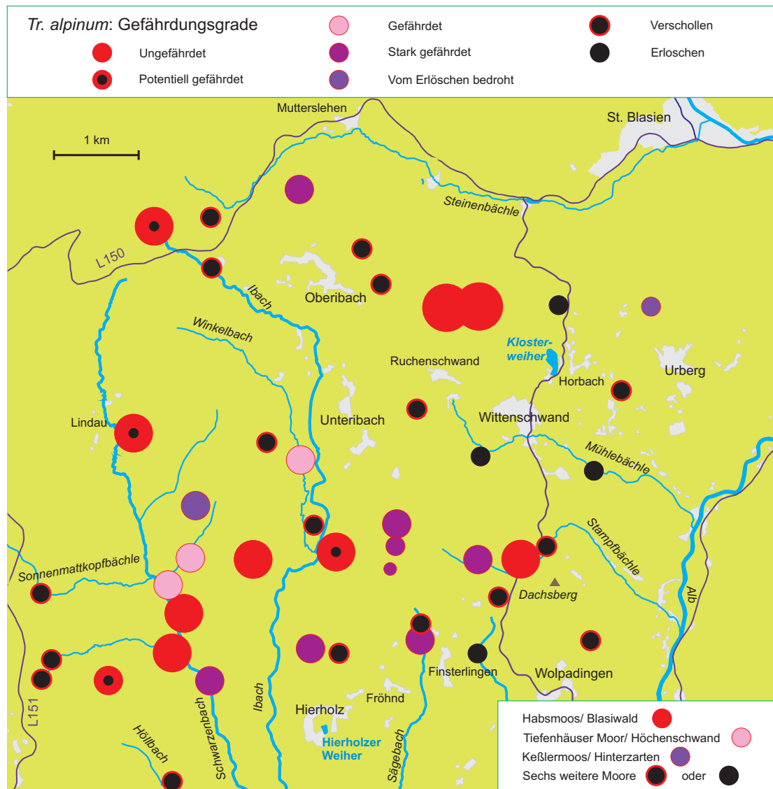
Abb. 5: Gefährdungsgrade der Wuchsorte bzw. Vorkommen des Alpen-Wollgrases.
