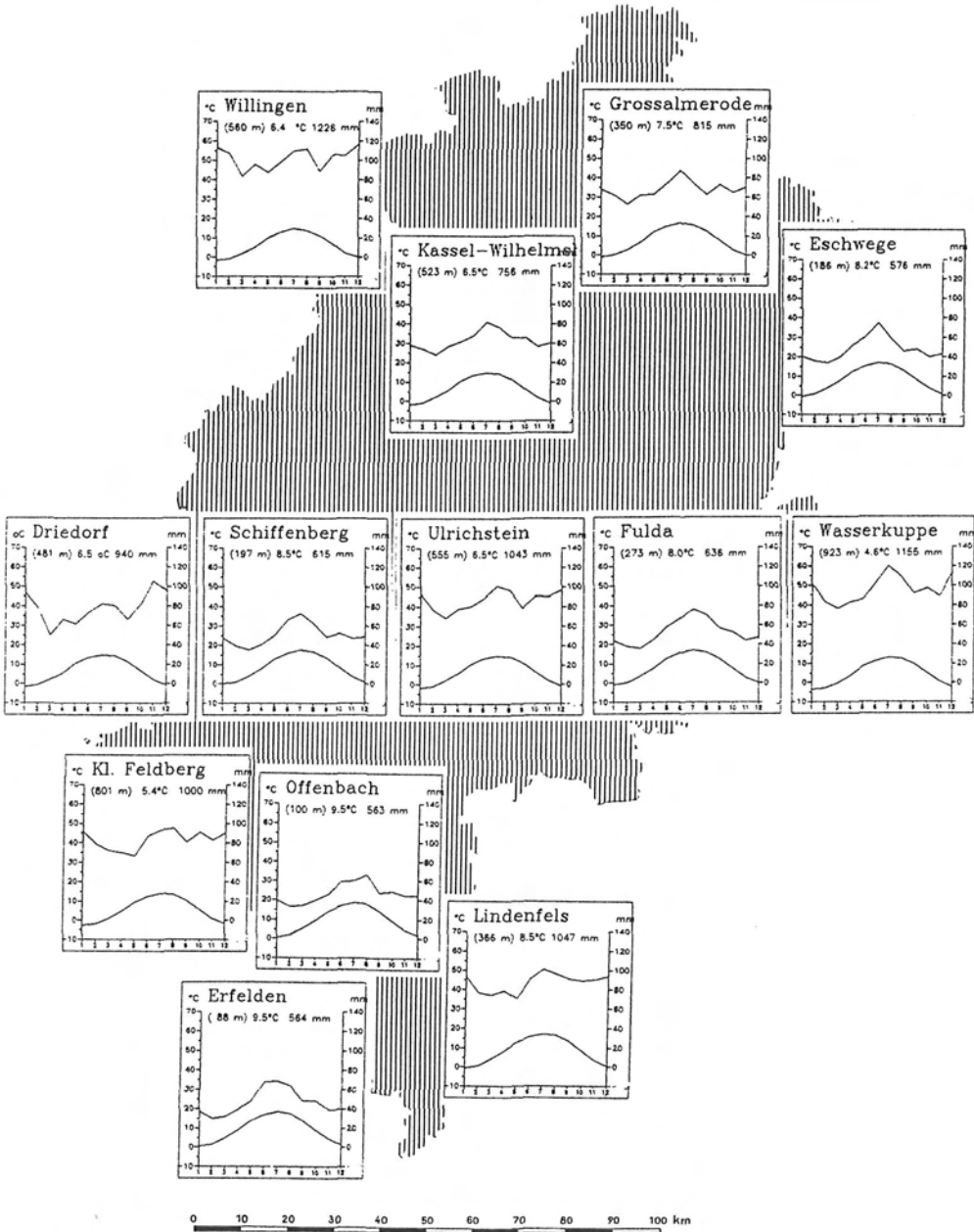
Abb. 3: Charakteristische Klimadiagramme
