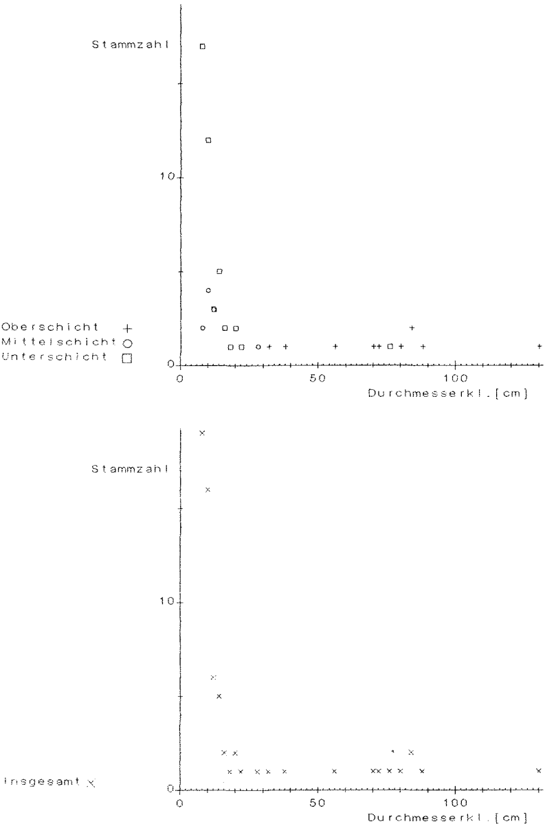
Abb. 44: Stammzahlverteilung, Probekreis 5 des NWR Karlsru rth
