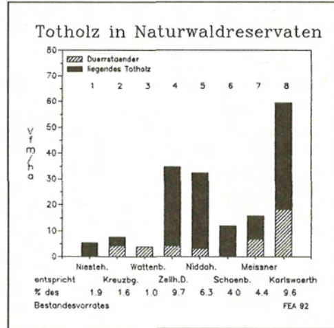
Abb. 57: Totholz in Naturwaldreservaten
