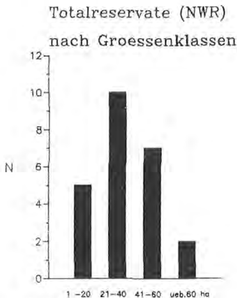
Abb. 14: Verteilung der NWR auf Größenklassen
