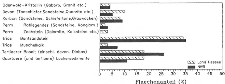
Abb. 9: Naturwaldreservatsflächen und Fläche des Landes Hessen, verteilt auf die geologischen Landschaften
