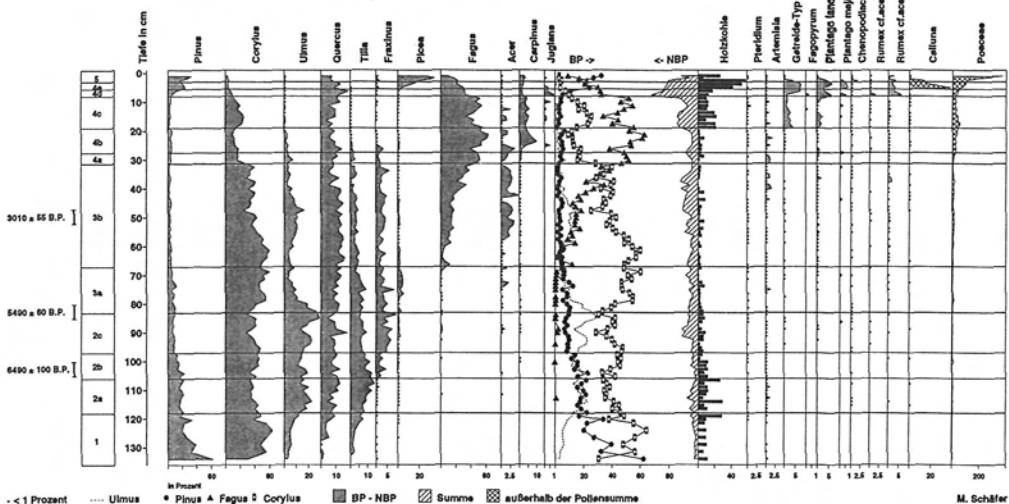
Abb. 22: Pollendiagramm Forellenteiche (vereinfacht). Pollenzonen: 1 Corylus-Pinus, 2a Ulmus-Tilia, 2b Ulmus-Corylus, 2c Ulmus-Fraxinus, 3a Corylus-Picea, 3b Corylus-Fagus, 4a Fagus-Quercus-Acer, 4b Fagus-Acer, 4c Fagus-Corylus, 4d Fagus-Quercus, 4e Fagus-Pinus, 5 Picea-Pinus.
