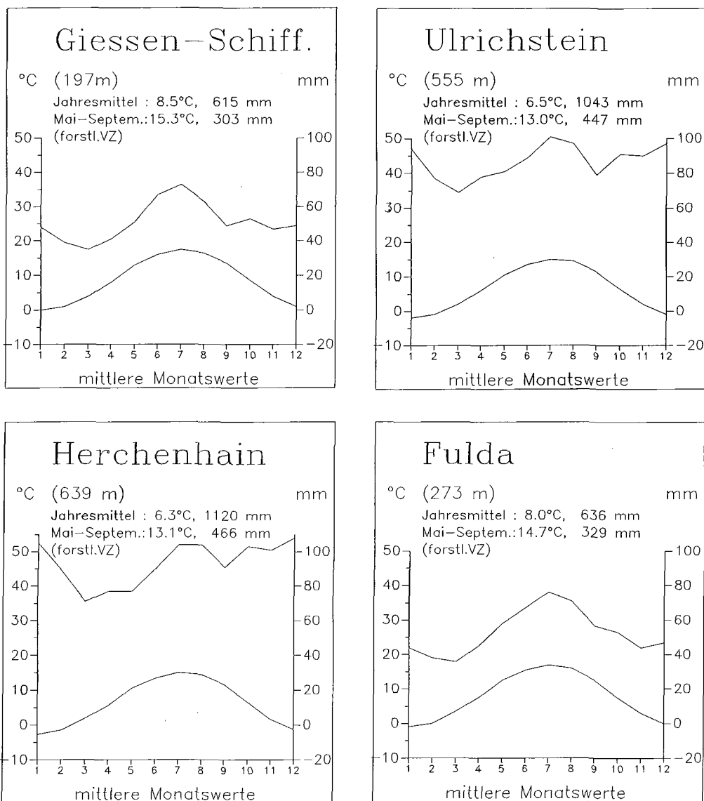
Abb. 6: Klimadaten der Beobachtungsperiode 1891 - 1955
