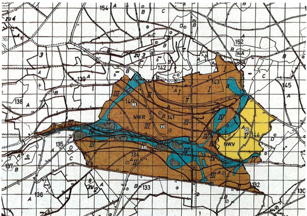
Karte 1: Substrat- und Bodentypen
