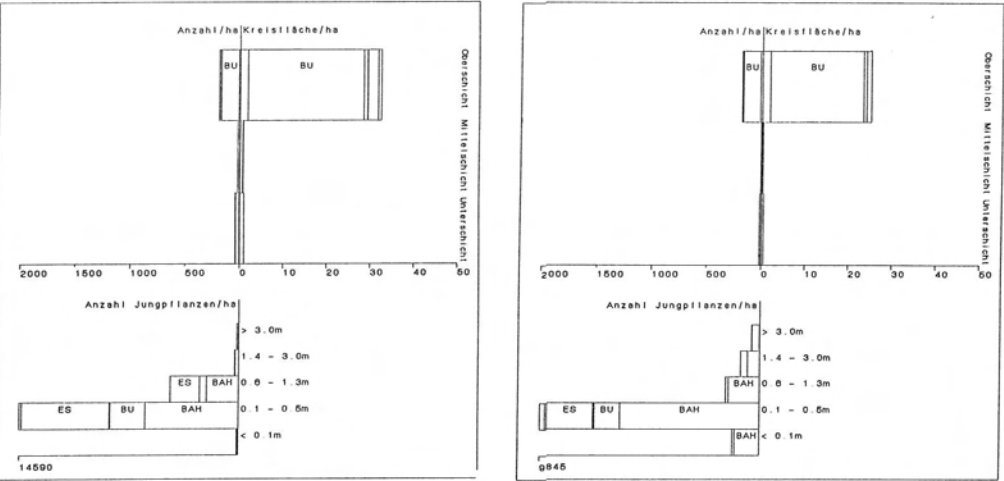
Abb. 28: Schematischer Bestandesaufriß mit Baumzahlen und Kreisfläche und Verjüngung nach Höhenklassen (links NWR, rechts NWV)
