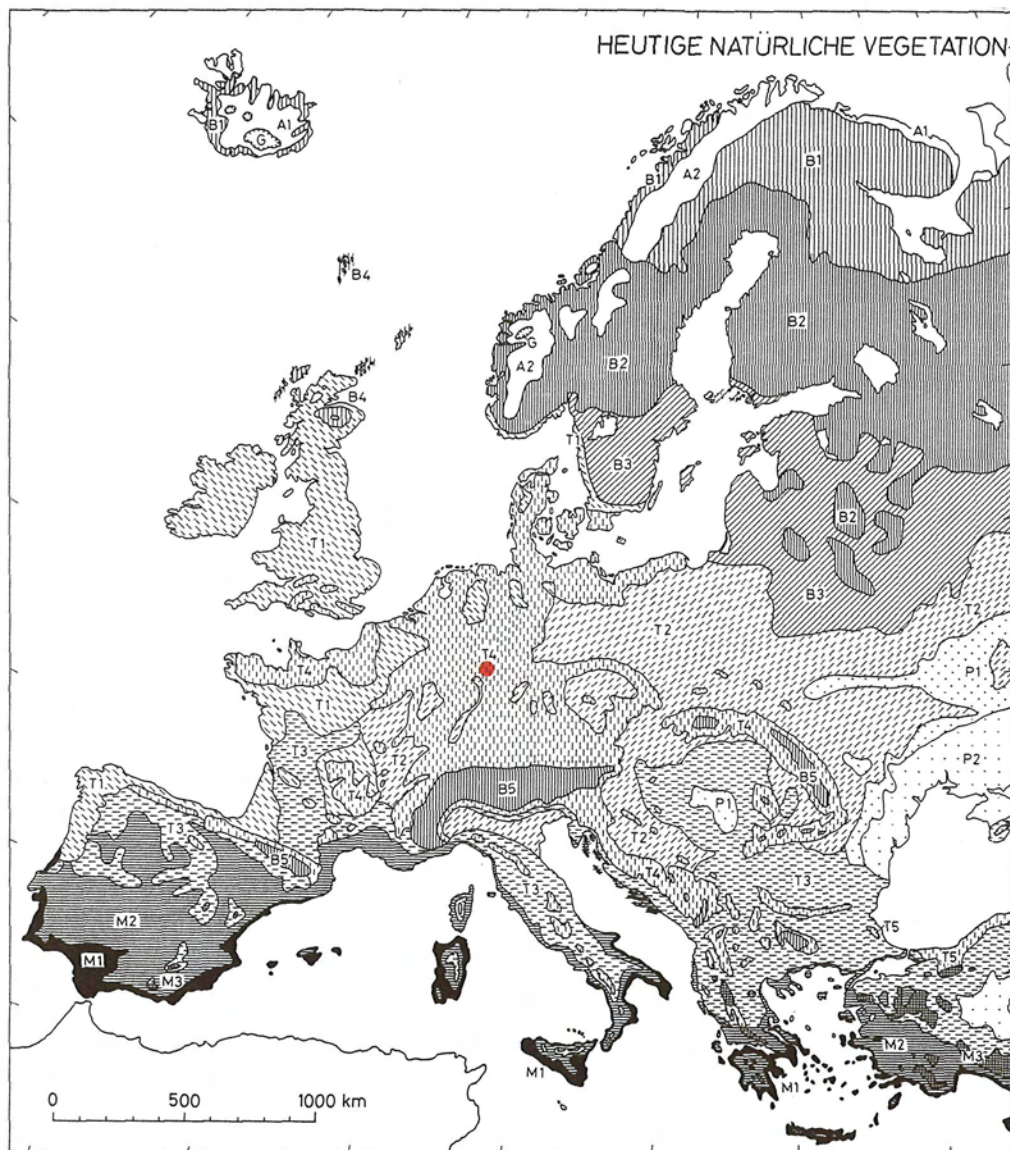
Abb. 3: Rotbuchenwälder (Bereich T4) aus LANG 1994 nach BOHN. Vogelsberg durch roten Punkt angedeutet.
