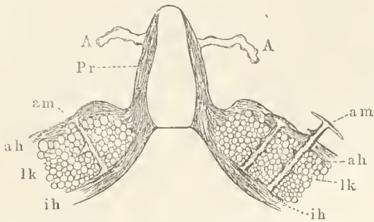
Medianer Schnitt durch das Porusrohr (Pr) und die Kapselwand der Gemmula. Vergr. etwa 250 fach. A Anhänge des Porusrohrs (Pr), am Amphidiskiden, ah äußere, ih innere Kapselhülle, lk die dazwischen gelegene Luftkammerschicht.
