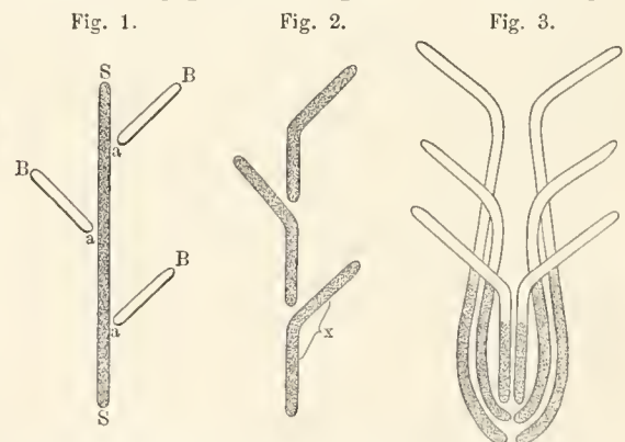
Fig. 1. Schema des Aufbaues der höheren Pflanzen nach Caspar Friedrich Wolff. S = Stengel, B = Blätter, a = Ansatzstellen der letzteren an dem Stengel. — Fig. 2. Schema des Aufbaues der höheren Pflanzen nach Goethe. x ist eine Einheit, bestehend unten aus Stengel, oben aus Blatt. — Fig. 3. Schema des Aufbaues einer höheren Pflanze nach Gaudichaud.
