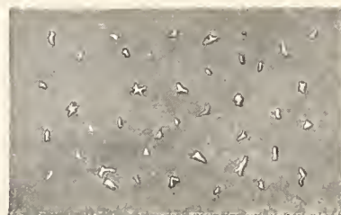
Aphanizomenon flos aquae . Schwebekörper, nach längerem Liegen der Zellen in 10 proz. Kalisalpetrolösung durch Druck isoliert. Vergrößerung etwa 700.
