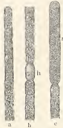
Aphanizomenon flos aquae Ralfs. a einzelner Faden, dessen Zellen mit in der Figur hell erscheinenden Schwebekörpern erfüllt ist; b derselbe mit einer Heterocyste h, welche nur 2 Schwebekörper enthält; c einzelner Faden mit einer Spore s, die keine Schwebekörper, wohl aber reichlich Körnchen anderer Art enthält. Vergrößerung etwa 700.
