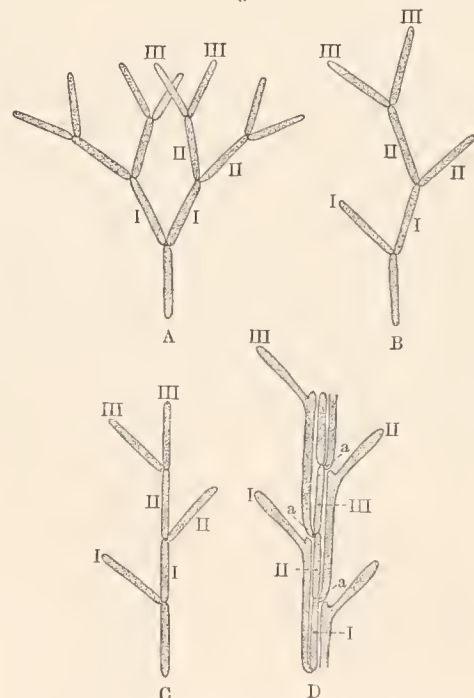
Fig. 4. Phylogenetische Entwicklung einer höheren Pflanze D aus einer Gabel-Alge A nach Ansicht des Verf. a die ursprünglichen Ansatzstellen der Urblätter.
