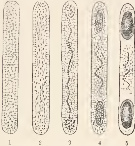
1 2 3 4 5 Sporenbildung bei Bacillus Bütschlii Schaudinn. (Nach der Tötung und Färbung mit Hämatoxylin.)
