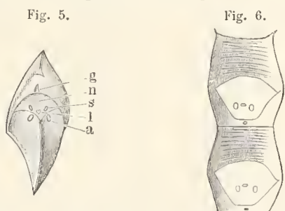
Fig. 5. Lepidodendron-Blattpolster in \frac{1}{2} . n = Blattnarbe, l = Leitbündelnarben, s = Seitennarben (Transpirationsstrangnarben), g = Ligulargrube, a = Transpirationsöffnungen. — Fig. 6. Ein Teil der Stammoberfläche einer Sigillaria mit zwei Blattnarben. Letztere zeigen ein Mittel- und zwei Seitennarben, entsprechend den in Fig. 5 mit l und s bezeichneten Narben. Über der Blattnarbe die Ligulargrube.
