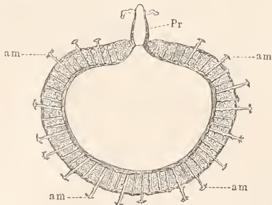
Medianer Längsschnitt durch die Gemmula ohne Inhalt. Vergr. 100 fach.
