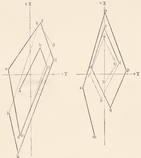
Fig. 5. Vektordiagramm.
