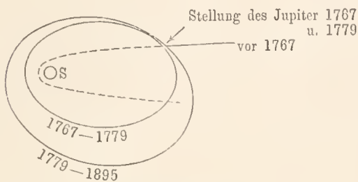
Bahn des Kometen Lexell.
