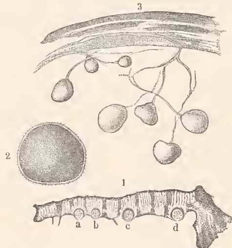
Fig. 1. Querschnitt durch einen Teil der Blattfieder. — Fig. 2. Einzelne Spore. — Fig. 3. Ein Teil der Wandung einer Höhlung mit einigen Sporen, die an Hyphen zu sitzen scheinen.
