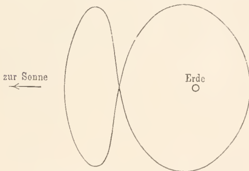
Mögliche Bahn eines Mondes nach Darwin.
