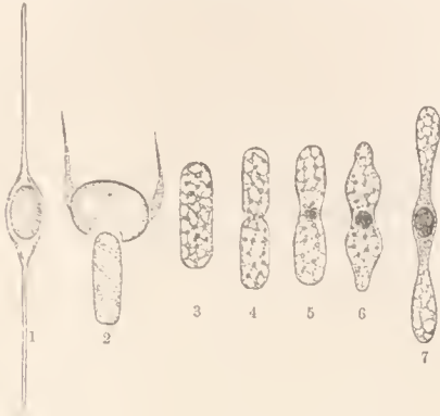
Sporenbildung bei Bacillus sporonema . Nach der Tötung und Färbung mit Eisenhämatoxylin.
