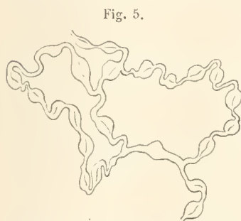
Digitalis purpurea. Tangentialschnitt von Faserzellen einer aufgesprungenen Anthere.
