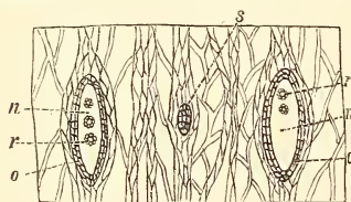
Fig. 2. Tangentialschnitt durch die äussere Rinde. Vergr.
