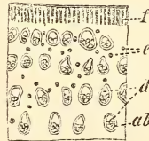
Fig. 3. Myelopteris radiata REN. Horizontalschnitt nat. Gr.
