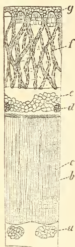
Fig. 1. Horizontalabschnitt von Sigillaria spinu- losa (denudata). Vergr.
