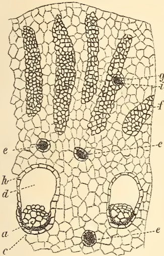
Fig. 2. Myelopteris radiata REN. Horizontalschnitt. Vergr.
