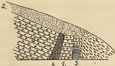
1. Nummulitenkalk. 2. Hangende Sandsteine. 3. Dunkle, sandig-glimmerige Schieferthone. 4. Kluftausfüllung.
