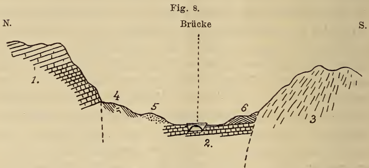
Im N. die Kalkmauern an der Dimbovitschora (1). Im S. die Kalke in der Enge der Dimbovitza. (3.) 2. Die Kalkscholle im Grunde des Thalkessels. 4. Mergelschiefer mit Sandstein-Einlagerungen. 5. Mürbe, rundhöckerige Sandsteine. 6. Sandsteine mit Mergelschiefer-Einlagerungen.
