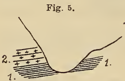
1. Nummulitenkalkmergel. 2. Festere Nummulitenkalke.
