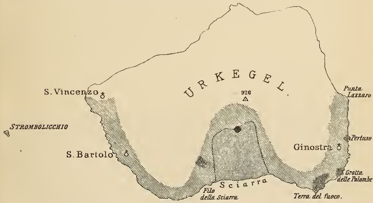
Petrogr. - Geolog. Skizze des Vulkans.
