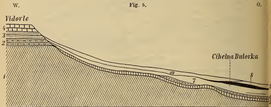
Uebersichtliches Längsprofil von der Anhöhe „Vidovle“ zur Ziegelei Bulovka. 1. Silurschiefer d.; 2. Perutzer Schichten; 3. Korycaner Sandsteine; 4. Turoner Pläner; 5. zersetzter Schiefer; 6. schotterige Lage; 7. grauer Gelblehm; 8. dunkelbrauner Lehm; 9. graubrauner Gelblehm; 10. lichter Gelblehm.
