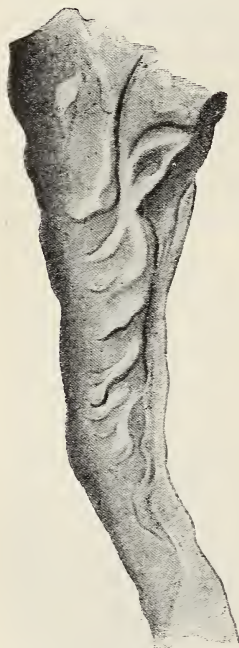
Fig. 1. Mit thoniger Substanz übersintertes Röhren im Lehm, sich nach oben theilend. Tübingen. 10:1.
