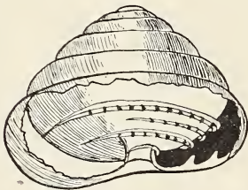
Fig. 1. Anordnung der Lamellen bei Strobilops labyrinthica (SAY).
