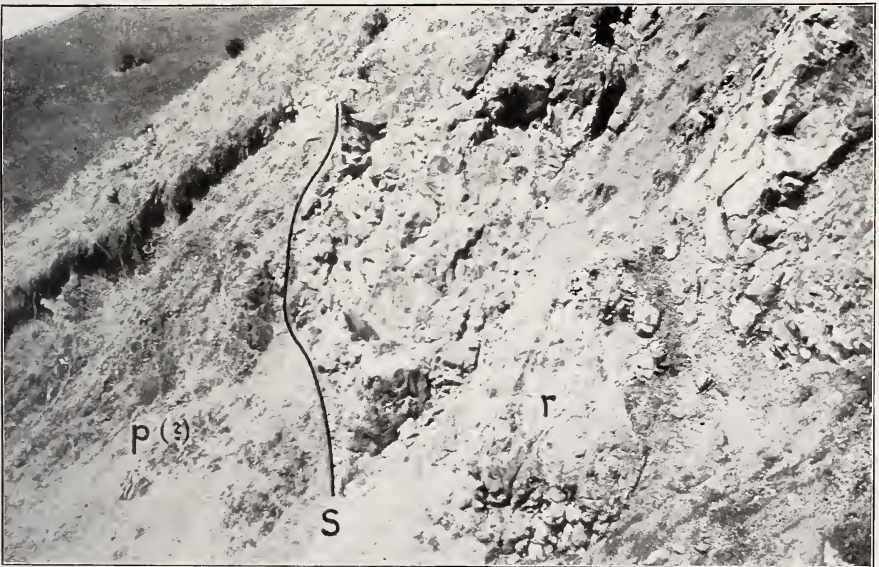
Fig. 2. Raiblerauschluß an der Mittenwalder Straße.
