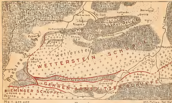
Geologische Kartenskizze des Wettersteingebirge, gez. von H. Mylius mit Benutzung der Karte von O.M.Reis.
