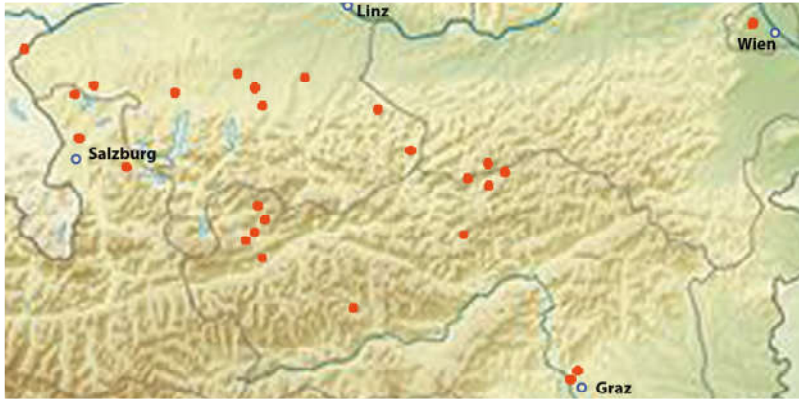
Abb. 1. Bythinella -Probestandorte
