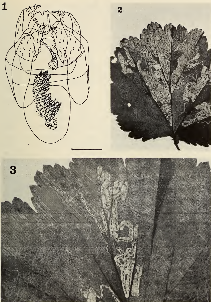
Abb. 1. Stigmella dryadella (HOFMANN), männl. Kopulationsapparat, Präp. Nr. 84/235/Hue., Brand Innertal 1100 m, ex 1. Dryas octopetala L., 10.8.1984 (Z 315). – Abb. 2 : Stigmella pretiosa (HEINEMANN), Minen an Geum rivale L., Brandnertal, Sonnenlagant Alpe 1300-1350 m, 14.9.1984 (Z 679). – Abb. 3 : detto, stärker vergrößert. Skala repräsentiert 0,1 mm.
