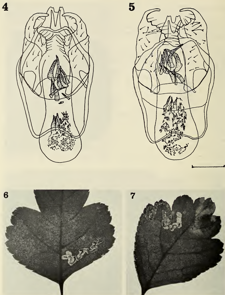
Abb. 4. Stigmella pretiosa (HEINEMANN), männl. Kopulationsapparat, Präp. Nr. 84/108/Hue., Brandnertal, Lünerkrinne 2100 m, ex 1. Geum montanum L., 27. 2.1984 (Z 129). – Abb. 5 : Stigmella pretiosa (HEINEMANN), männl. Kopulationsapparat, Präp. Nr. 84/104/Hue., Brandnertal, Sonnenlagant Alpe 1350 m, ex 1. Geum rivale L., 4.10.1984 (Z 652). – Abb. 6 : Stigmella crataegella KLIMESCH, Mine an Crataegus oxyacantha L. em. JACQ., Brandnertal, Bürserberg Tschappina 900-950 m, M.8.1984 (Z 611). – Abb. 7 : Stigmella oxyacanthella (STANTON), Mine an Crataegus oxyacantha L. em. JACQ., Feldkirch-Gisingen Ardetzenberg 450 m, E.9.1984 (Z 737). Skala repräsentiert 0,1 mm.
