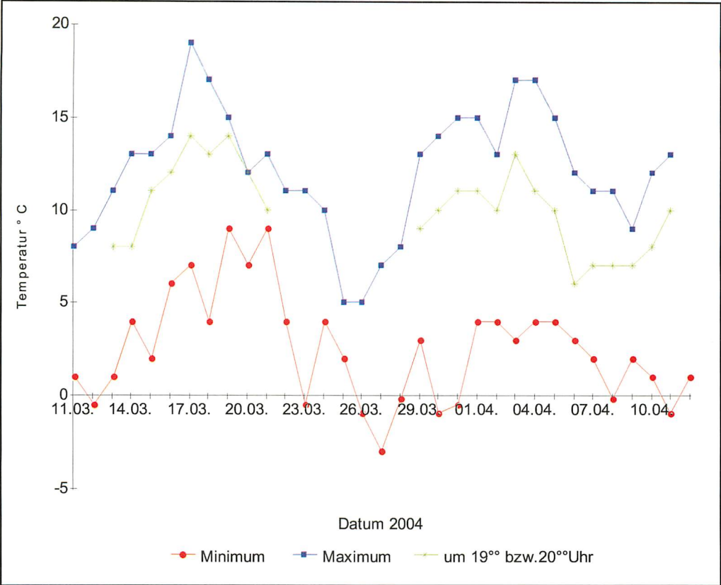
Abb. 14. Temperaturverlauf während der ersten Freßzeiten und des Nachwinterschlafs 2004; neben dem Minimum und dem Maximum des Tages ist auch die für die Jagdmöglichkeit wichtige Dämmerungstemperatur (vor und nach Anordnung der Sommerzeit) teilweise berücksichtigt.
