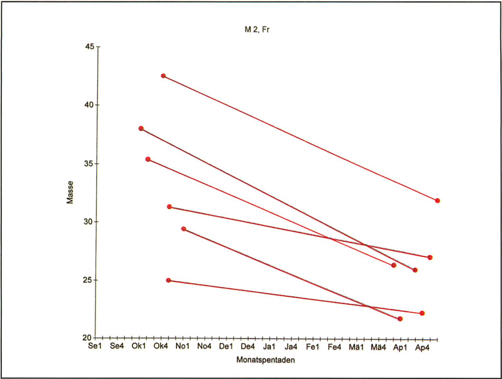
Abb. 10. Masseunterschied zwischen Herbst und Frühjahr bei 6 Abendseglermännchen, verschiedene Jahre
