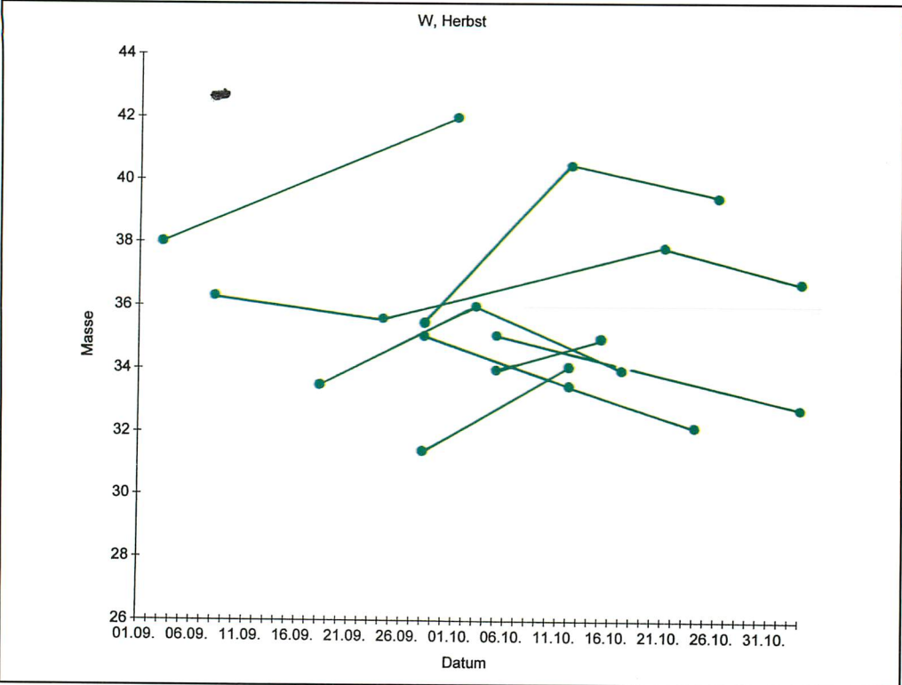
Abb. 8. Entwicklung der Körpermasse von 8 Abendseglerweibchen im Herbst, verschiedene Jahre
