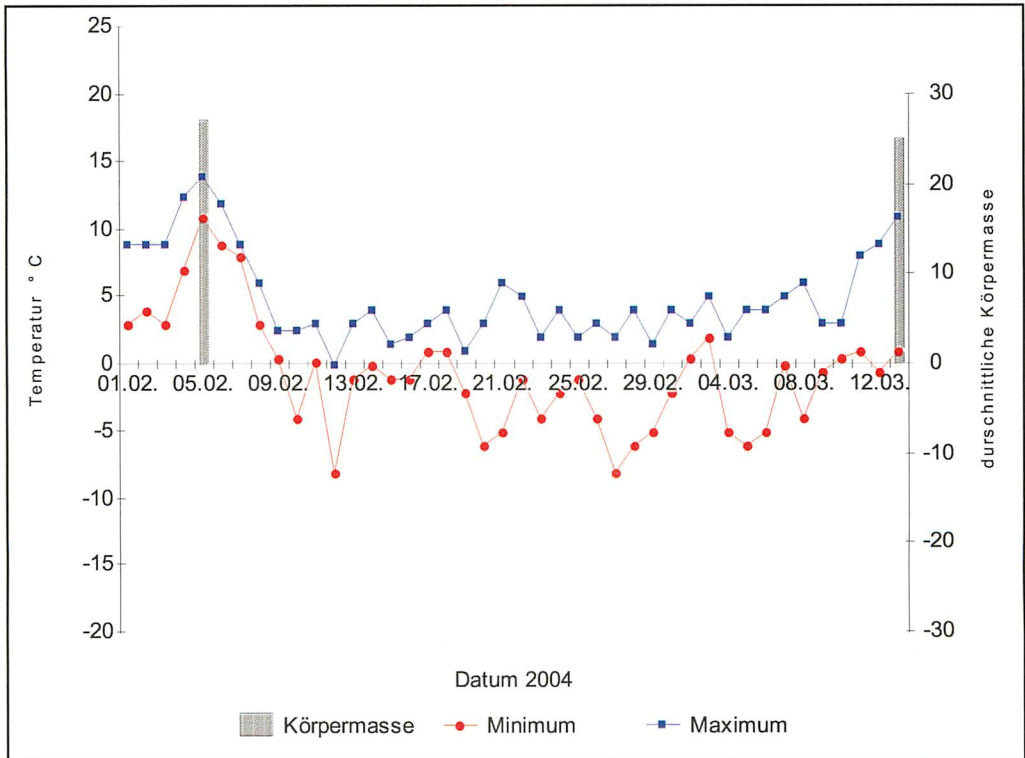
Abb. 13. Temperaturverlauf im Februar und März 2004 (Ortsrand von Beeskow) während des Aufenthaltes der Frühtückkehrer und Durchschnittsmasse der angetroffenen Abendseglergruppen
