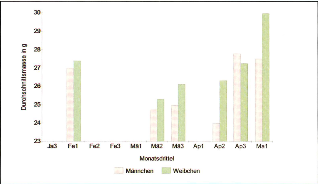
Abb. 15. Körpermasseentwicklung von Abendseglern während wechselhafter Möglichkeiten zum Jagdflug am Anfang des Jahres 2004
