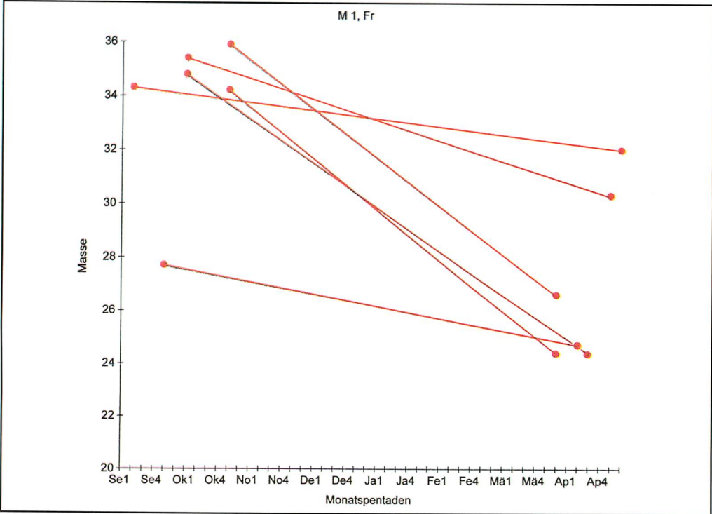
Abb. 9. Masseunterschied zwischen Herbst und Frühjahr bei 6 Abendseglermännchen, verschiedene Jahre
