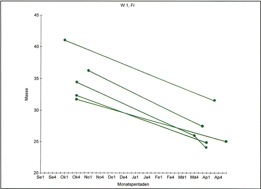
Abb. 11. Masseverlust zwischen Herbst und Frühjahr bei 5 Abendseglerweibchen, verschiedene Jahre
