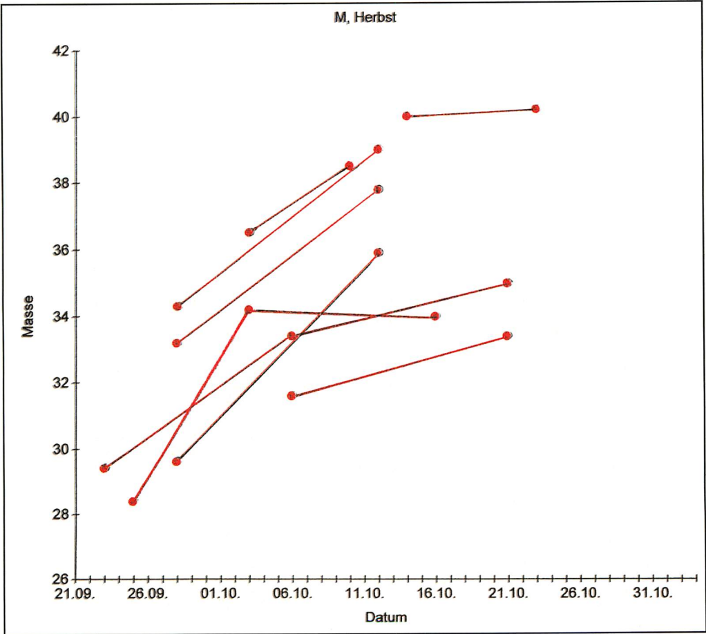
Abb. 7. Masseentwicklung von 8 Abendseglermännchen im Herbst, verschiedene Jahre
