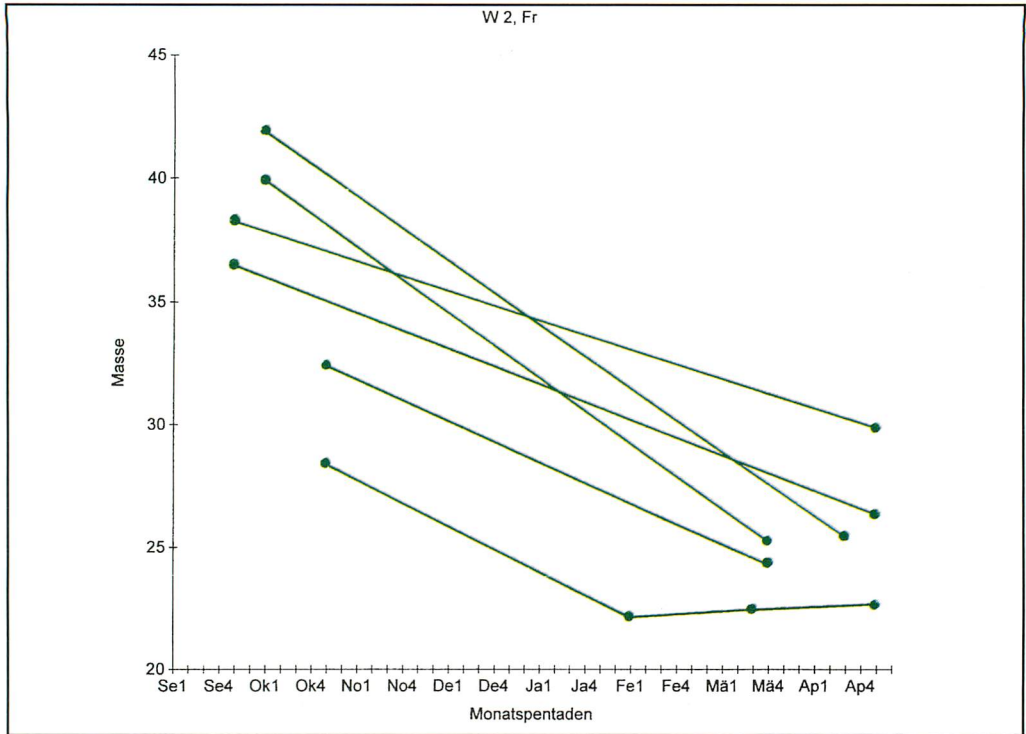
Abb. 12. Masseverlust zwischen Herbst und Frühjahr bei 6 Abendseglerweibchen, verschiedene Jahre
